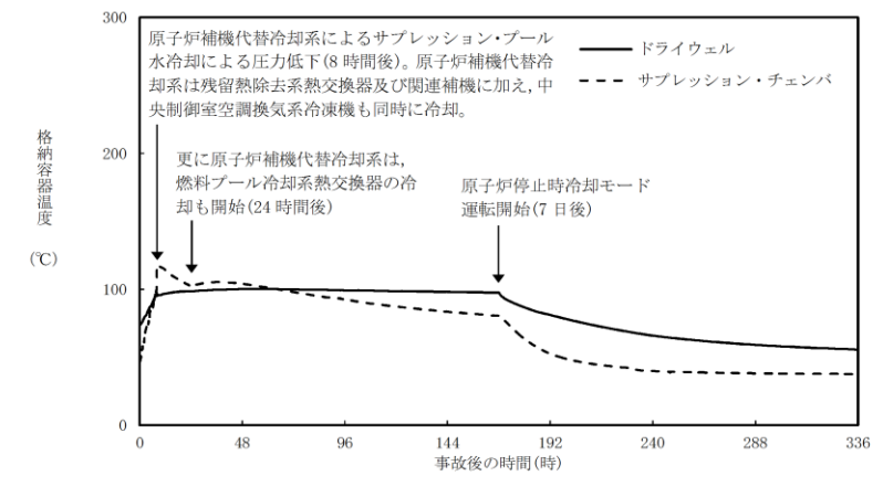
図 1.11 格納容器温度の推移
