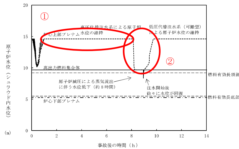
第 2.3.2-5 図 原子炉水位 (シユラウド内水位) の推移
