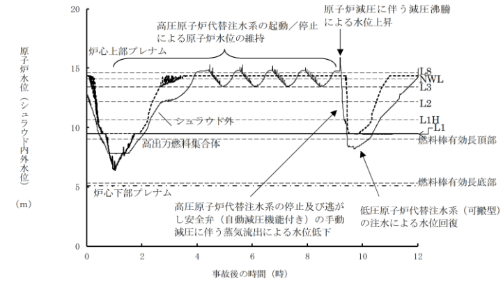
第 2.3.2.3-1(2) 図 事象発生 60 分後に注水を開始したケースにおける原子炉水位（シュラウド内外水位）の推移
