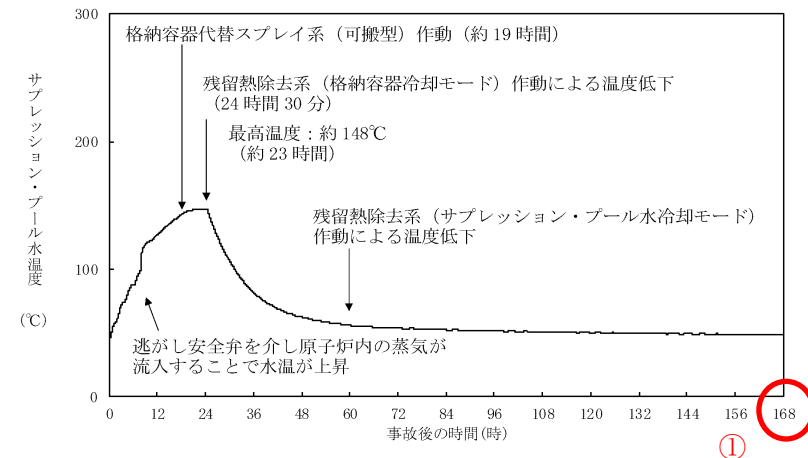
第 2.3.1.2-1(13) 図 サプレッション・プール水温度の推移
