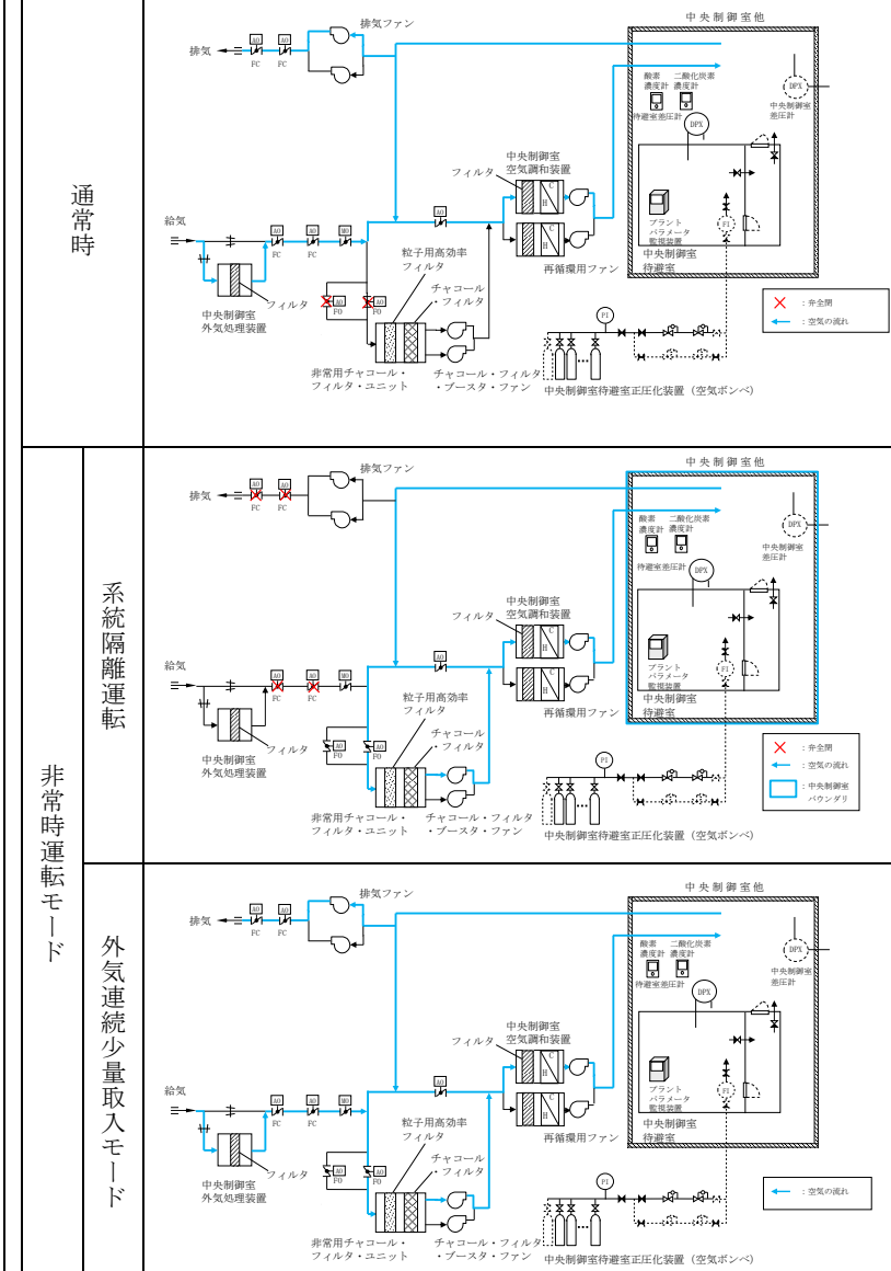
図4-2 2号炉中央制御室換気系の概要図
