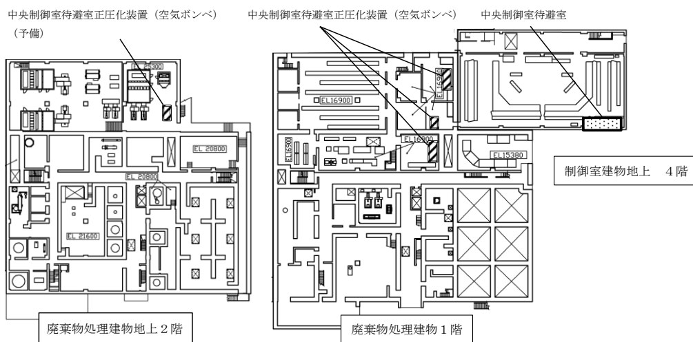
図 2.4-17 空気ポンペ設置 配置図
