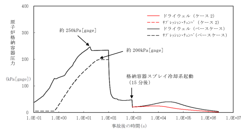
第4図 代替性確認評価ケース2とベースケースの評価結果比較 (原子炉格納容器圧力)
