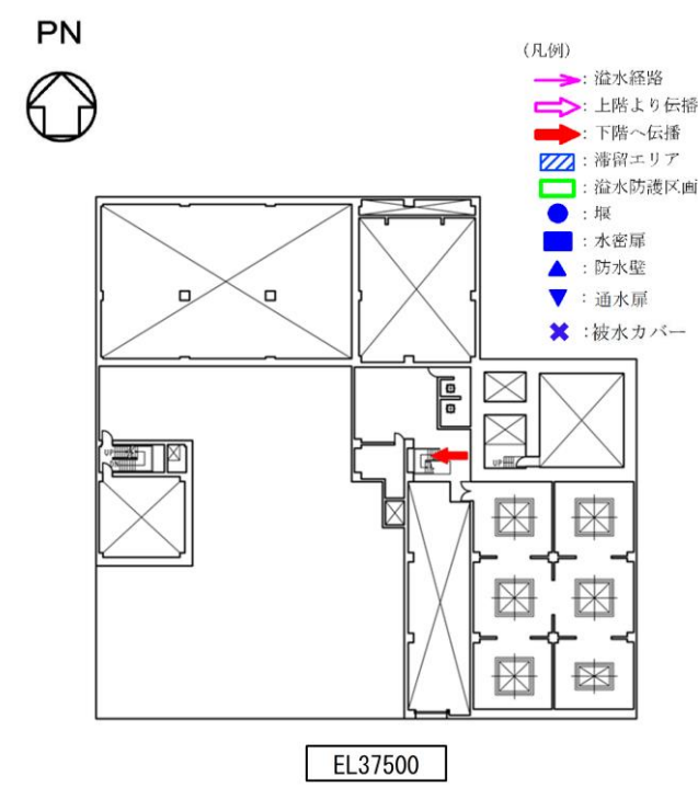
図 2-32 廃棄物処理建物 5階 溢水防護対策設備設置箇所
