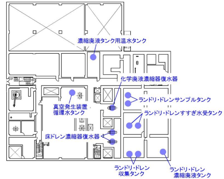
図 1-10 溢水源となり得る主な機器の配置 (廃棄物処理建物 3階 EL26.7m)
