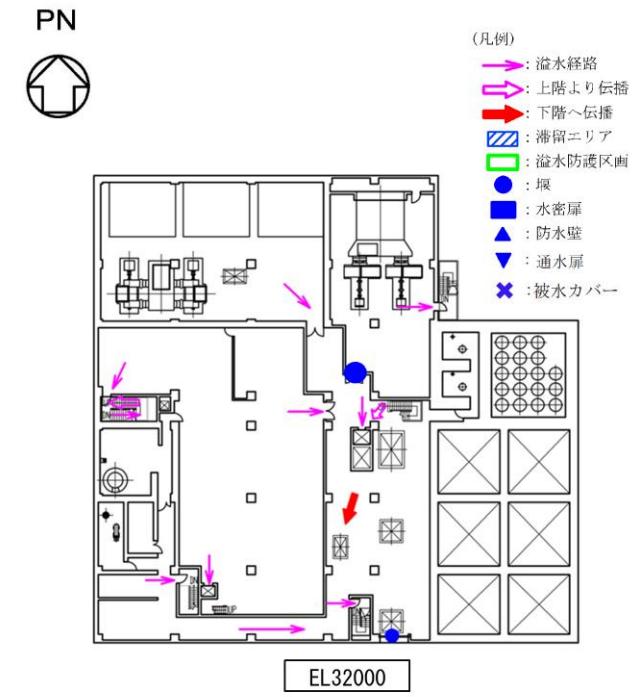
図 2-31 廃棄物処理建物 4階 溢水防護対策設備設置箇所
