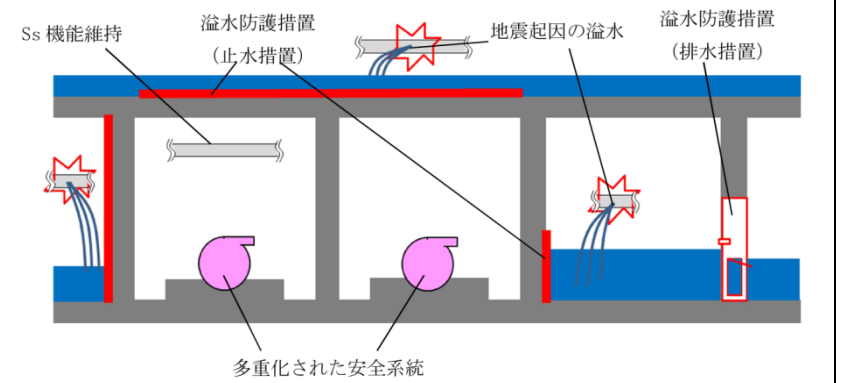
図1-3 地震起因の破損に対する溢水防護概念図
