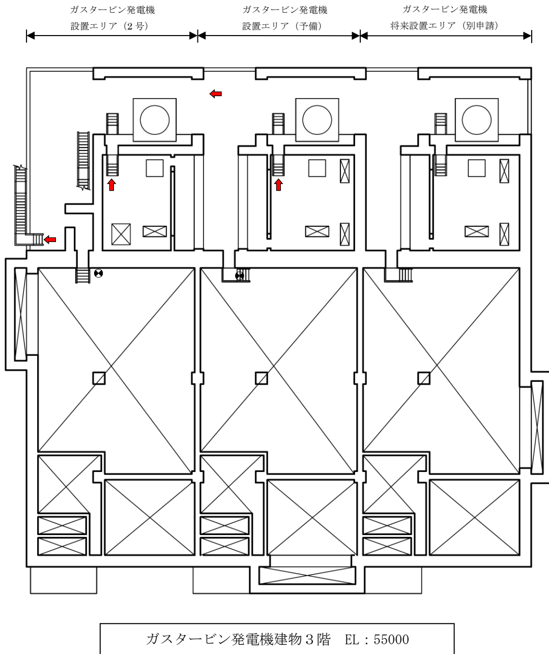
別紙2-2図 安全避難通路及び避難用の照明配置図
