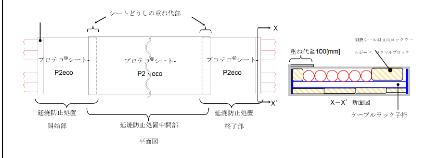
第1図 延焼防止シートの標準的な巻き付け方法（※の資料から抜粋）
