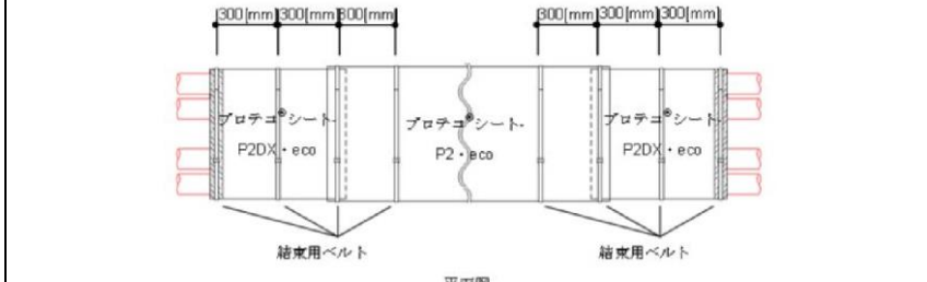
第2図 結束用ベルトの標準的な取付方法（※1 資料抜粋）
