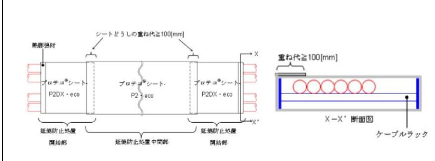
第1図防火シートの標準的な巻き付け方法（※1 資料抜粋）
