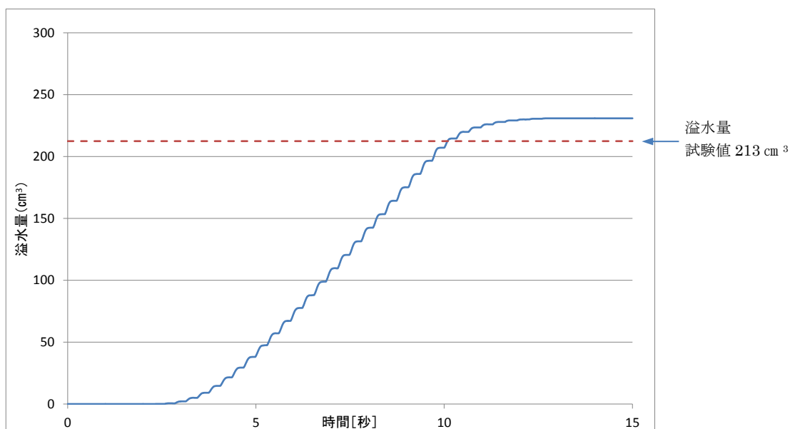
図 3-5 溢水量の解析結果
