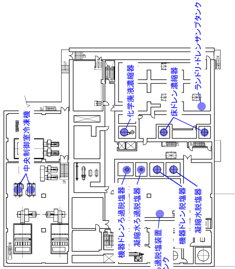
図 1-11 溢水源となり得る主な機器の配置 (廃棄物処理建物 2 階 EL22. 1m)
