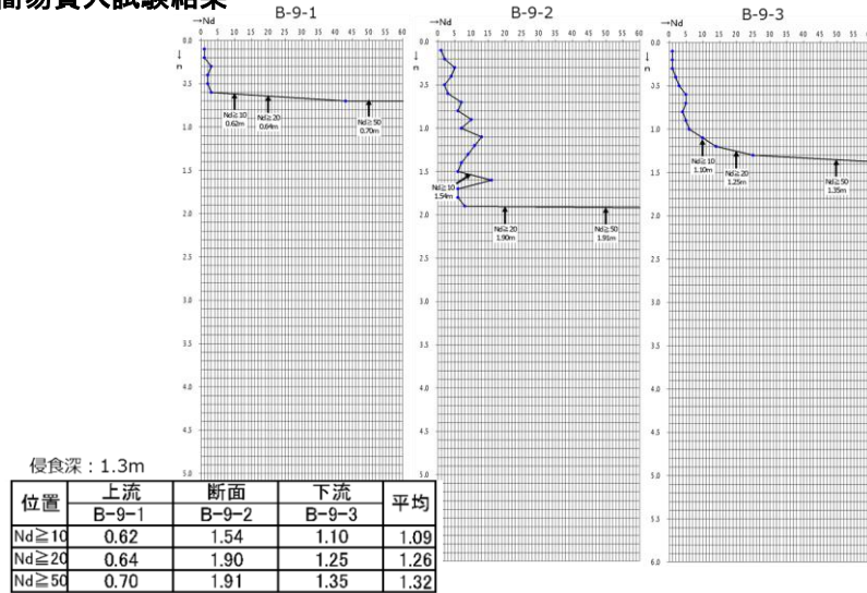
図-11 土石流危険溪流④の現地調査結果
