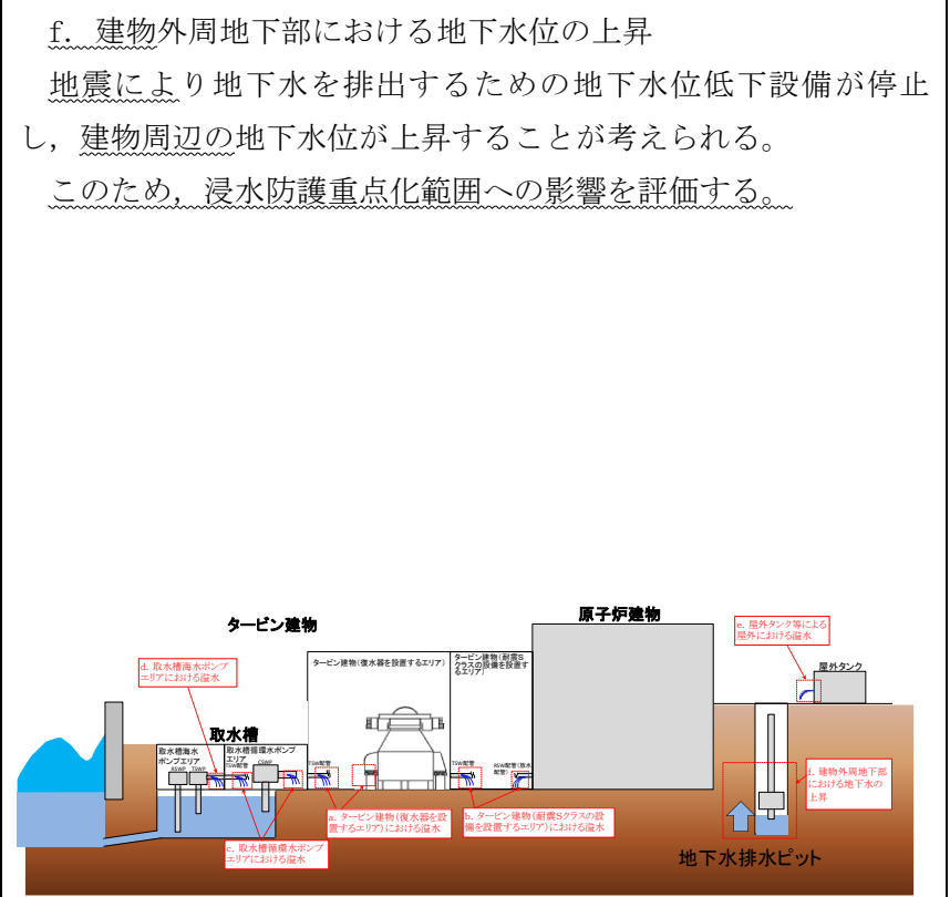
第2.4-4-1図 地震による溢水の概念図(低耐震クラスの機器及び配管の損傷)
