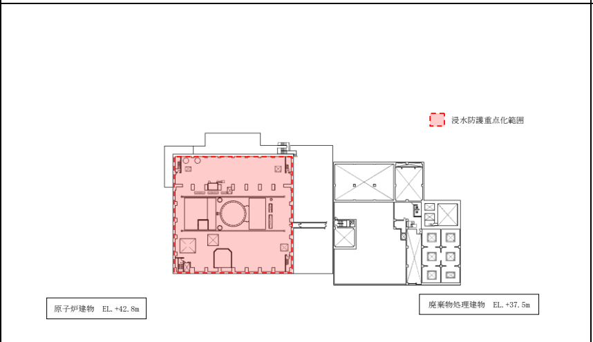
第2.4-2-4図 (5) 浸水防護重点化範囲 (断面図)
