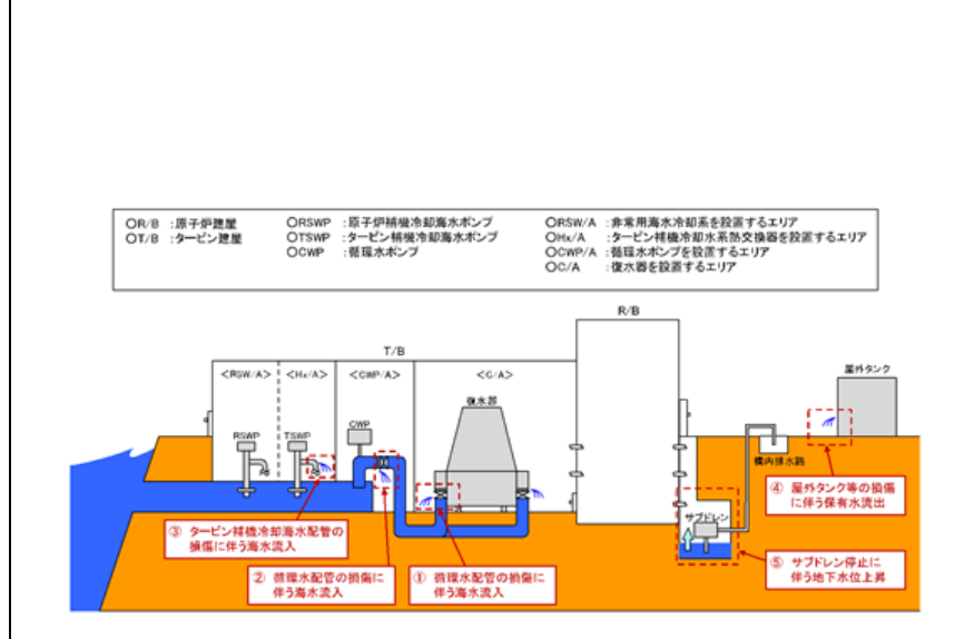
第2.4-3-1図 地震による溢水の概念図
