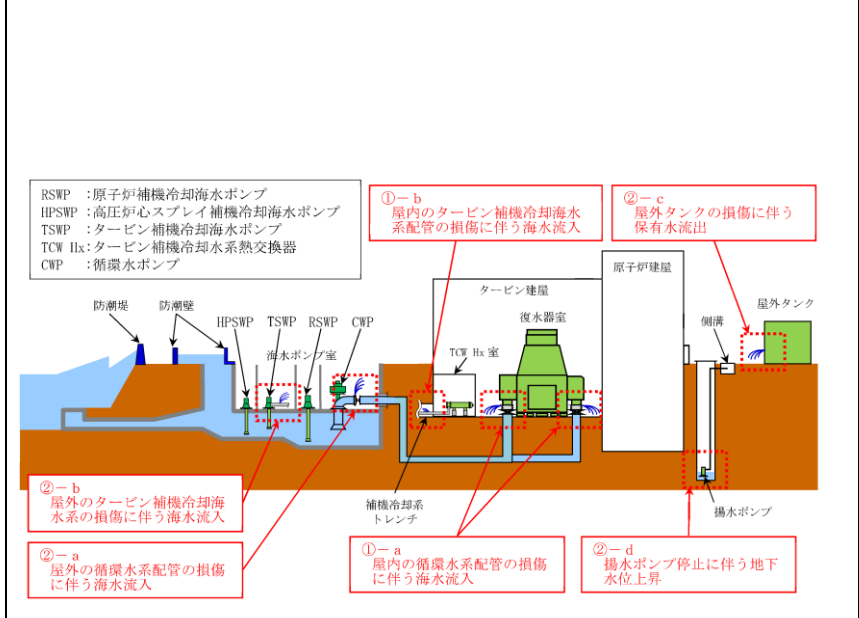
図2.4-6 地震による溢水の概念図
