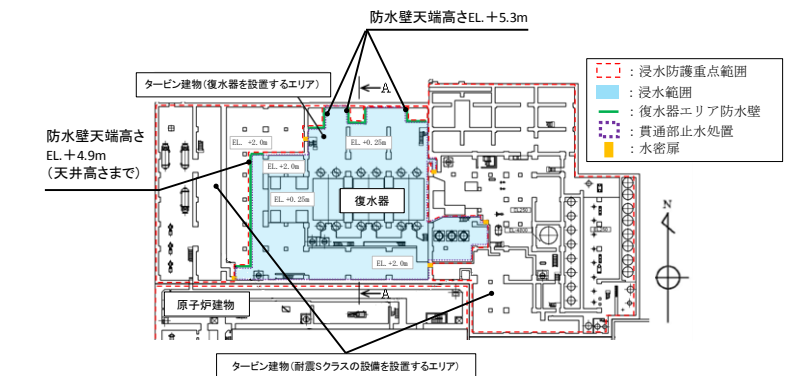
(平面図)
