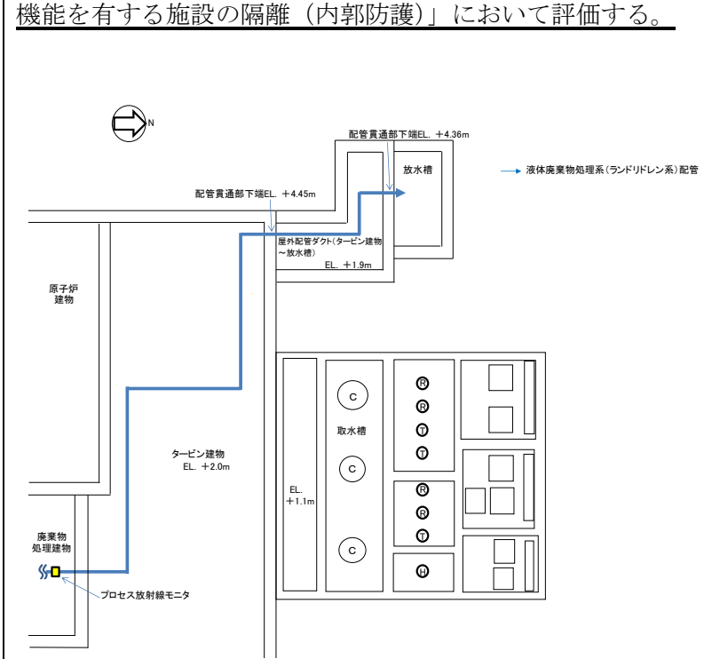
第2.2-16図 その他排水管の経路概要図
