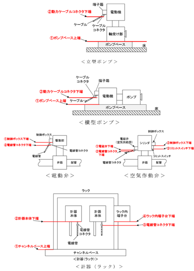
第2.3-10図各設備の機能喪失高さ概略図
