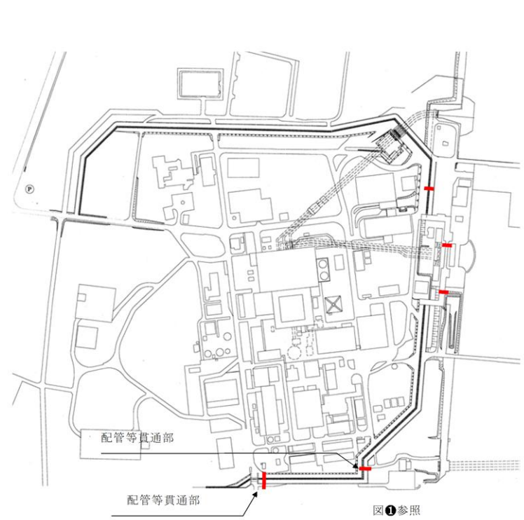
第2.2-43図 防潮堤貫通部配置図
