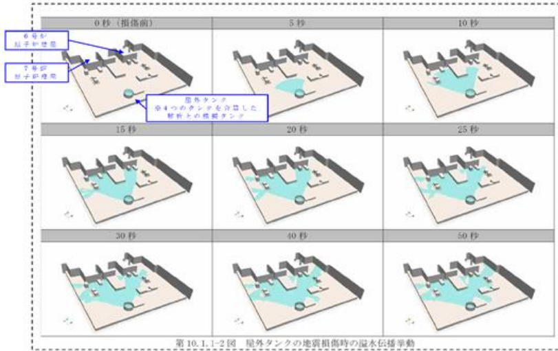
第2.4-7図 溢水伝播挙動のイメージ
