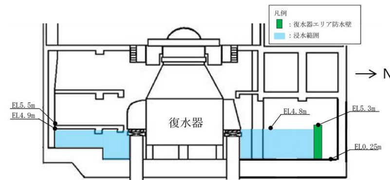
(A-A 断面)
