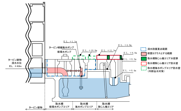
(断面図)
