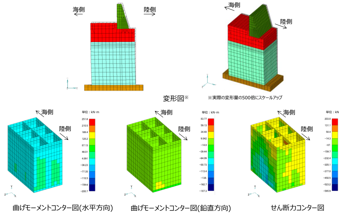
第 10-5-12 図 3次元静的 F E M解析結果（輪谷部）
