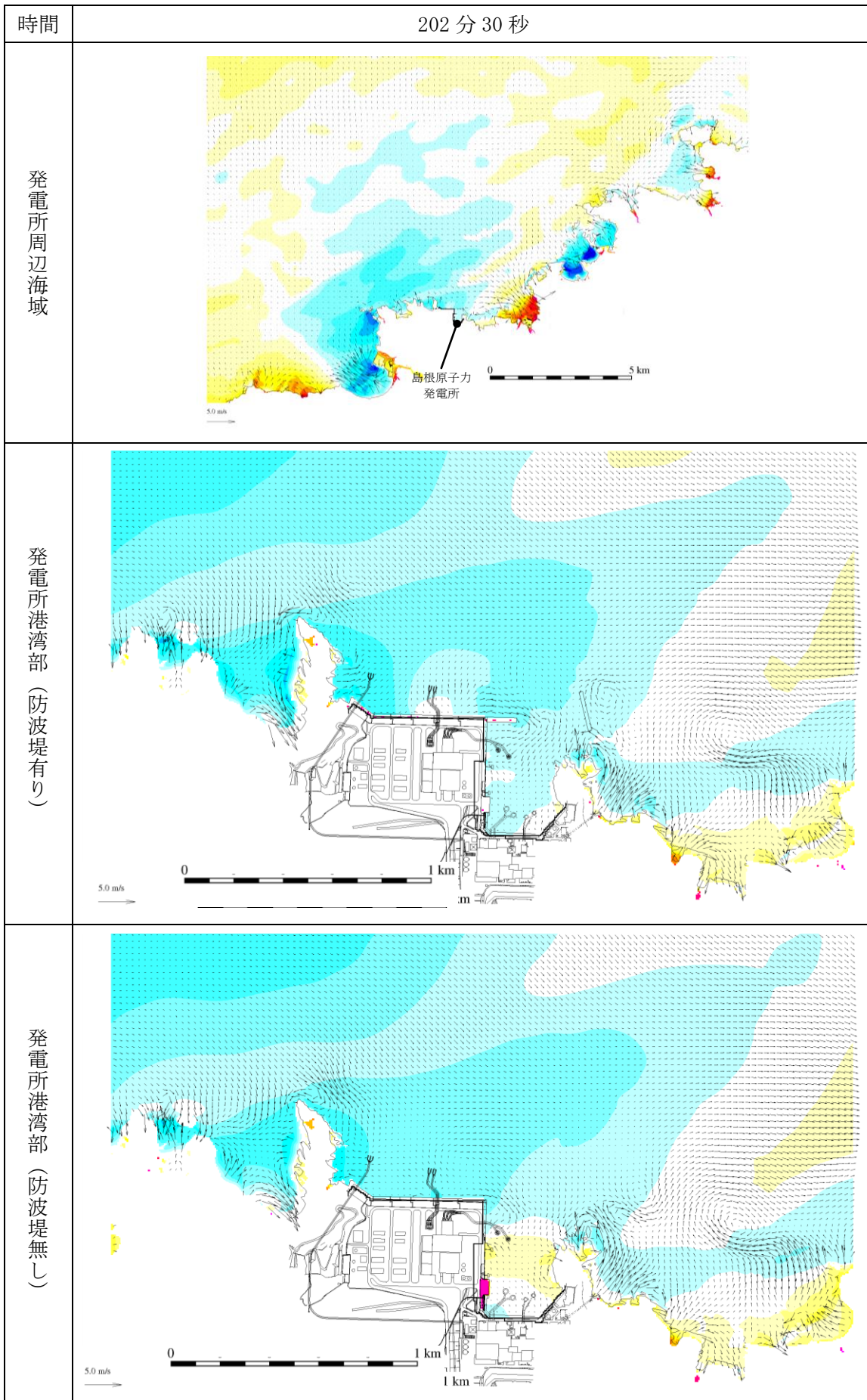
第 1 図 (206) 基準津波 1 の水位変動・流向ベクトル
