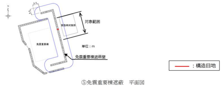
3-3-4 図 線状構造物の屈曲部及び隅角部
