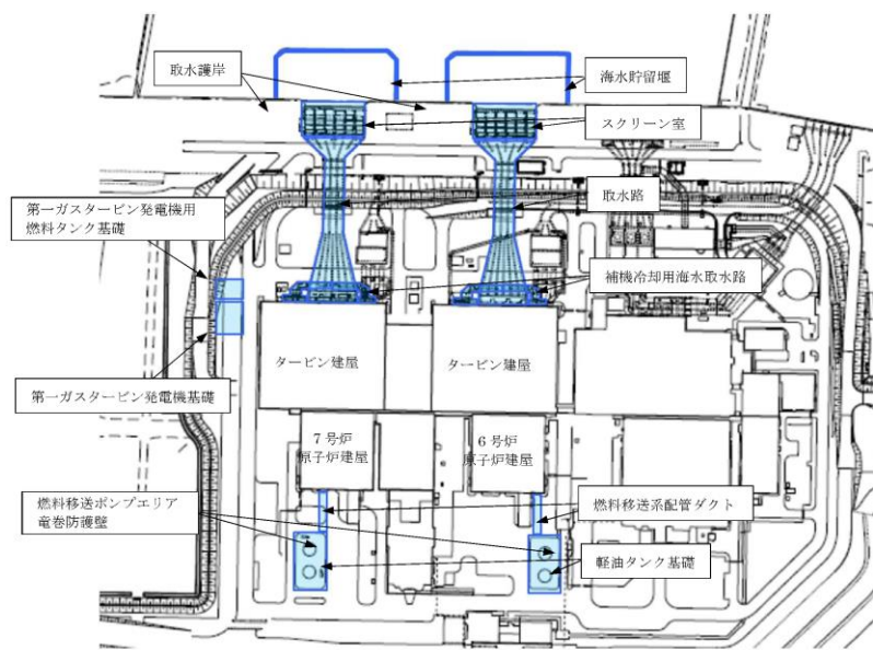
第3.3.4-1図 屋外重要土木構造物配置図
