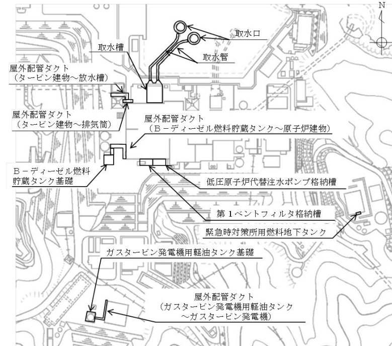
第3.3.4-1図 屋外重要土木構造物等配置図
