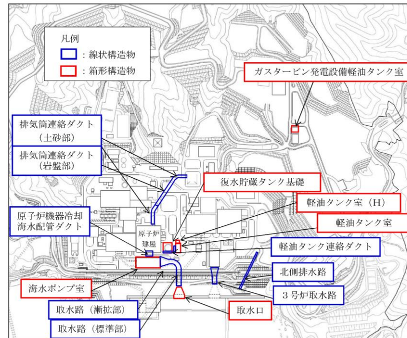
第3.3-4図 屋外重要土木構造物配置図
