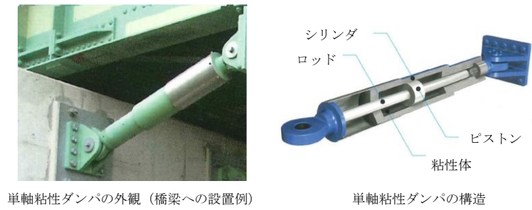
第 2-4 図 単軸粘性ダンパの外観及び構造
