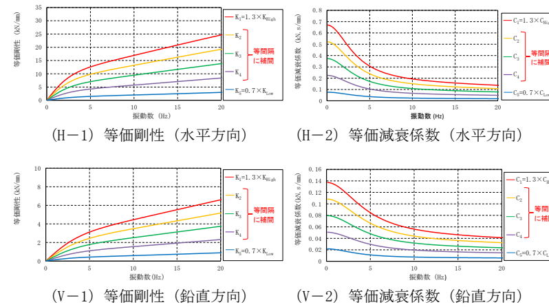
第 3-15 図 地震応答解析モデルにおける段階的な減衰性能の設定 (中型の例)
