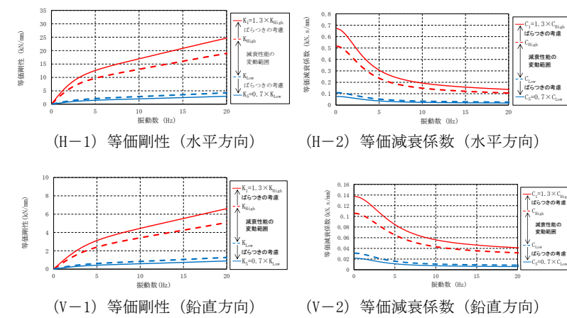
第 3-14 図 性能試験による減衰性能の上限と下限の設定 (中型の例)
