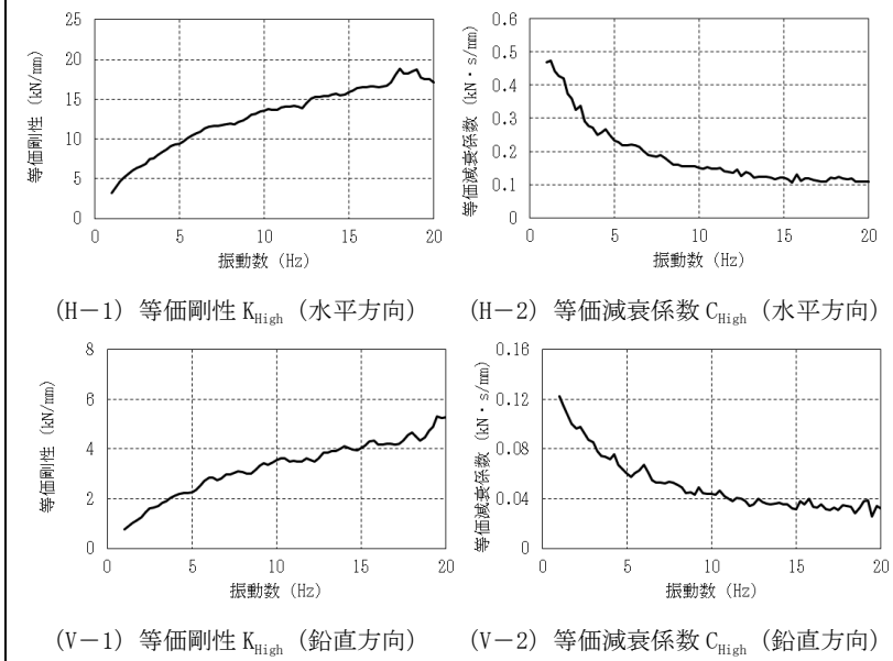
第3-9図 高側ダンパ試験性能 (中型の例)
