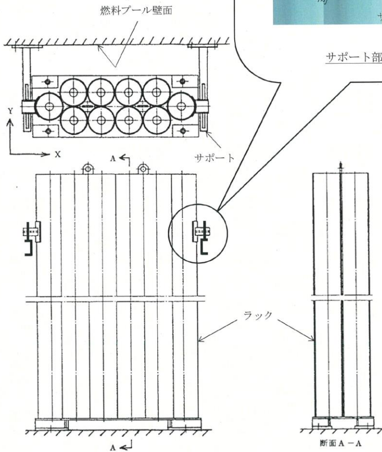
第3-1図 制御棒・破損燃料貯蔵ラック設置状態
