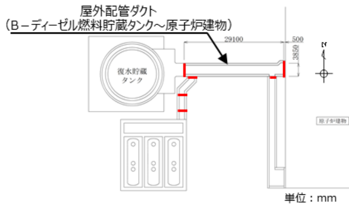
③ 屋外配管ダクト (B-ドイウム燃料貯蔵タンク～原子炉建物) 平面図
