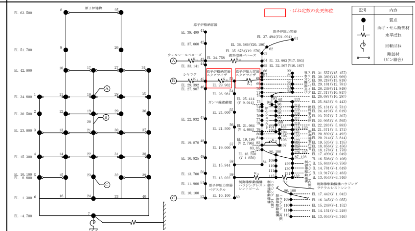
第1-2-1図 PCV-RPV-Rinモデル (NS方向)
