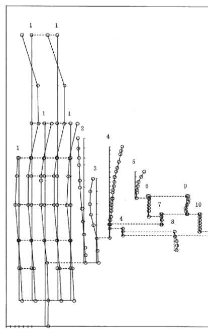
第2-2-9 図 (b) 今回工認モデル 第9次振動モード図 (NS方向)
