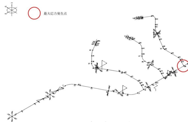
第6-8 図 給水系配管 (FDW-001 Aプラント)
