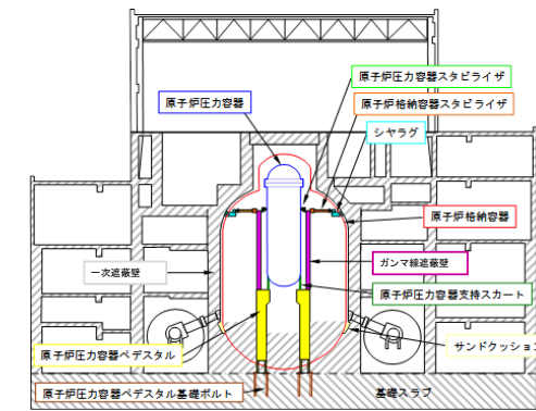
原子炉建物概略断面図
