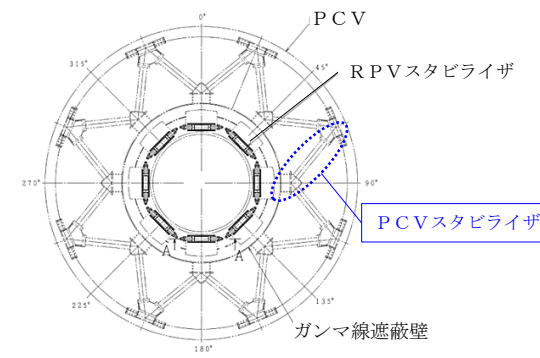
PCV平面図
