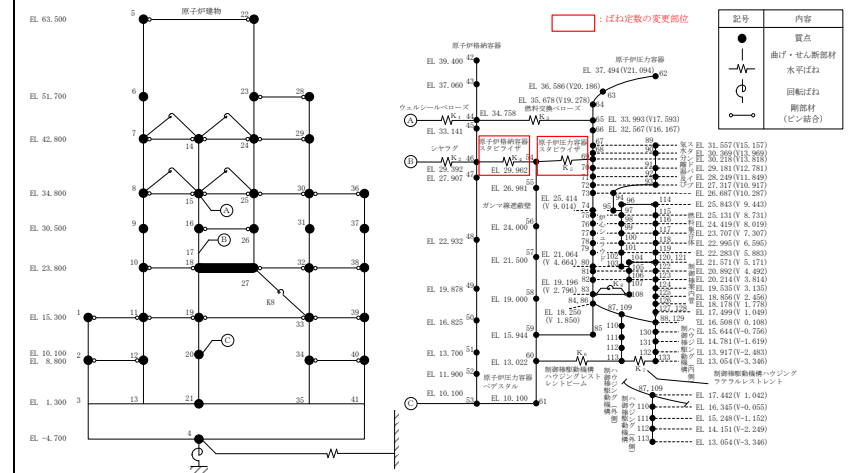
第1-2-2図 PCV-RPV-Rinモデル (EW方向)
