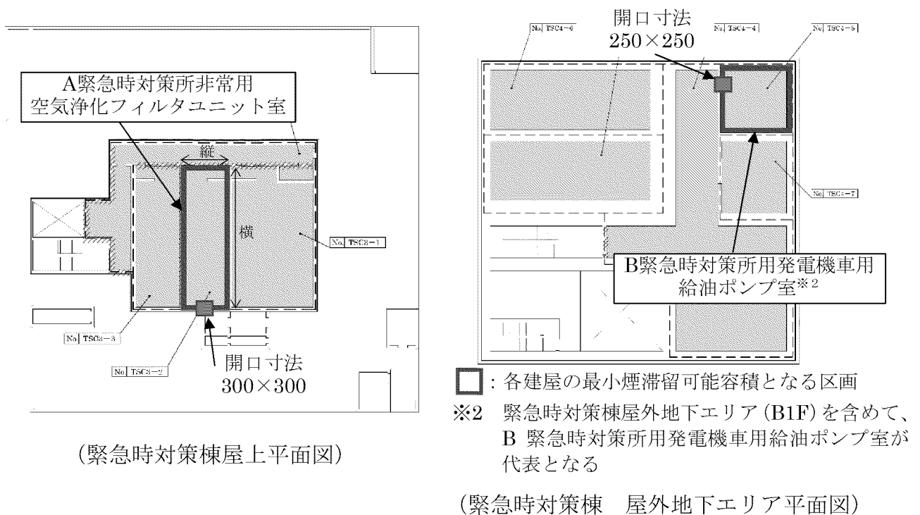
図 7-3 各建屋の代表区画の平面図
