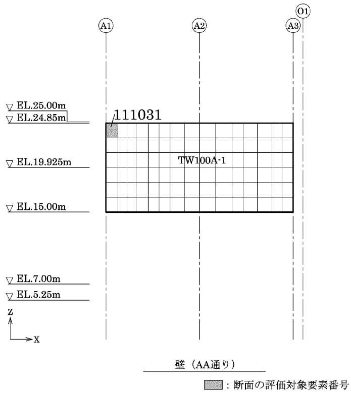
第 5-1 図 断面の評価対象要素番号(2/5)
