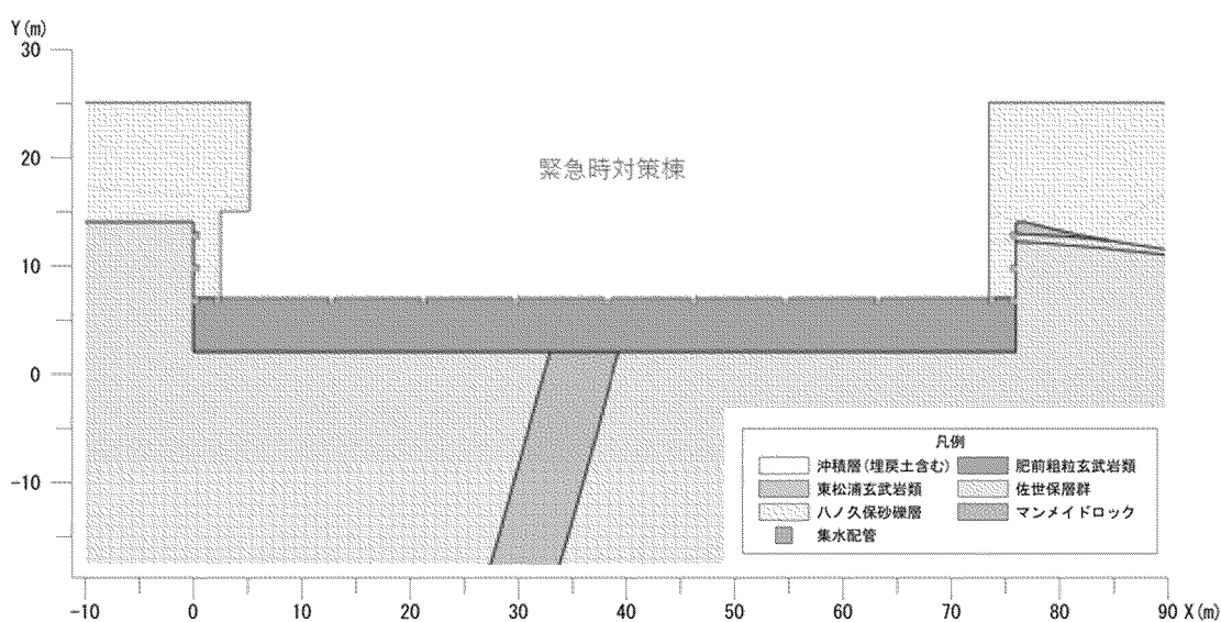
第 3 図 二次元浸透流解析モデル (X M -X M '断面) (拡大) (2/4)
