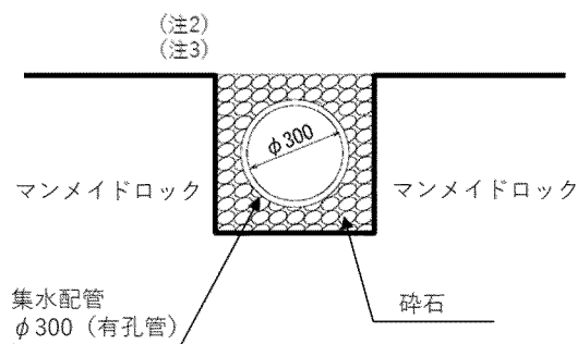
集水配管断面図
