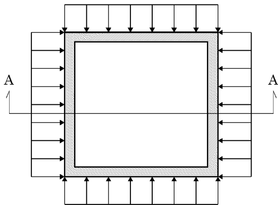
(a) 平面図
