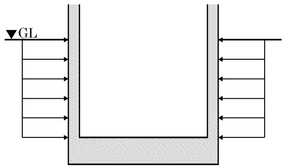
地震荷重加力方向
