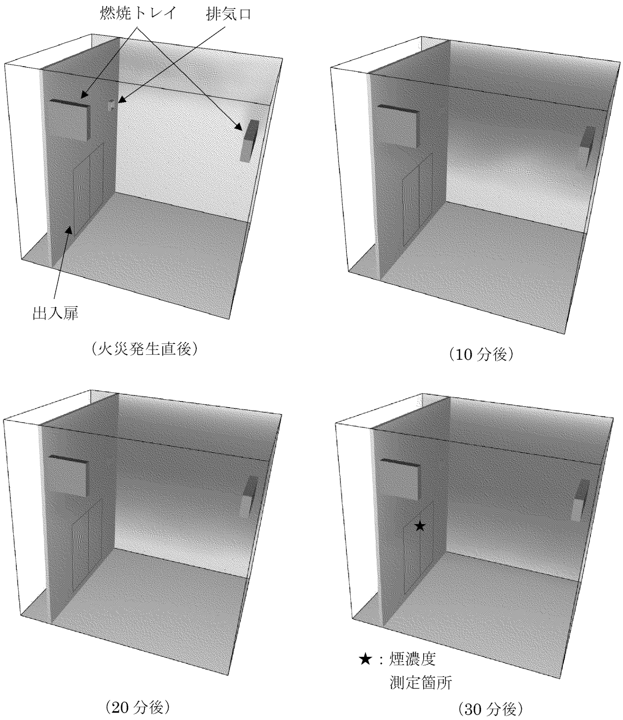
図 7-3 煙の流動状況結果
