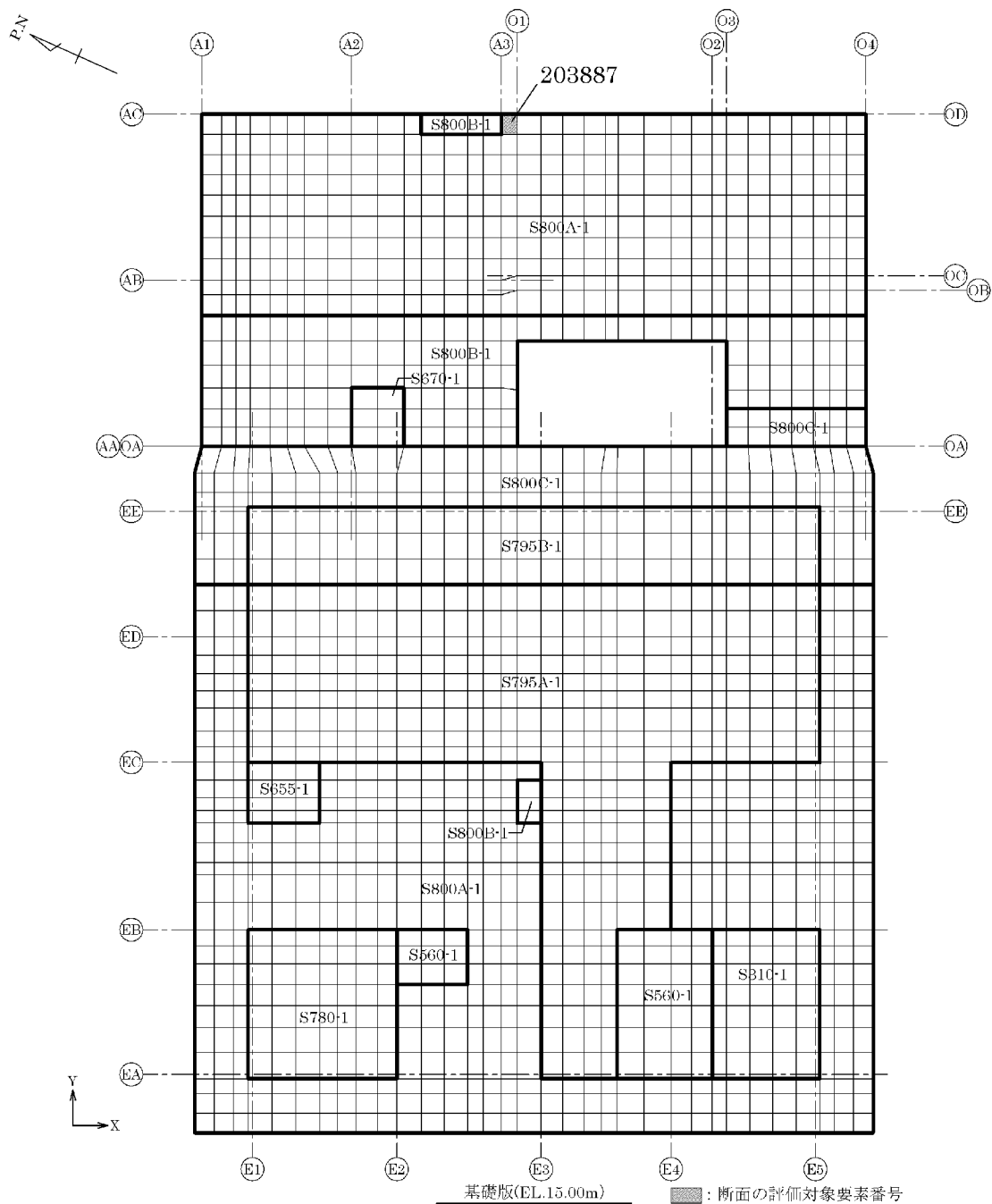
第3-1図 断面の評価対象要素
