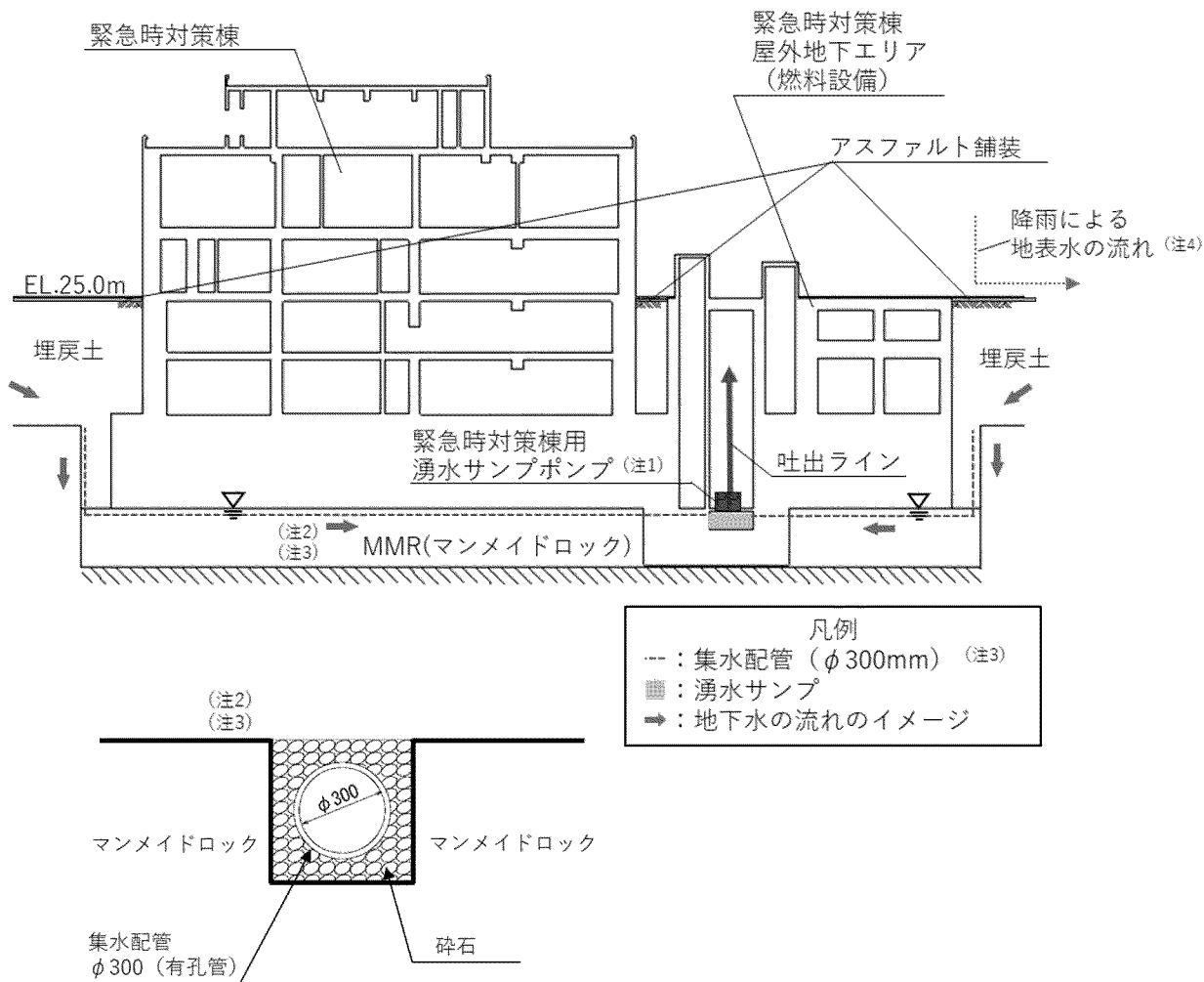
集水配管断面図
