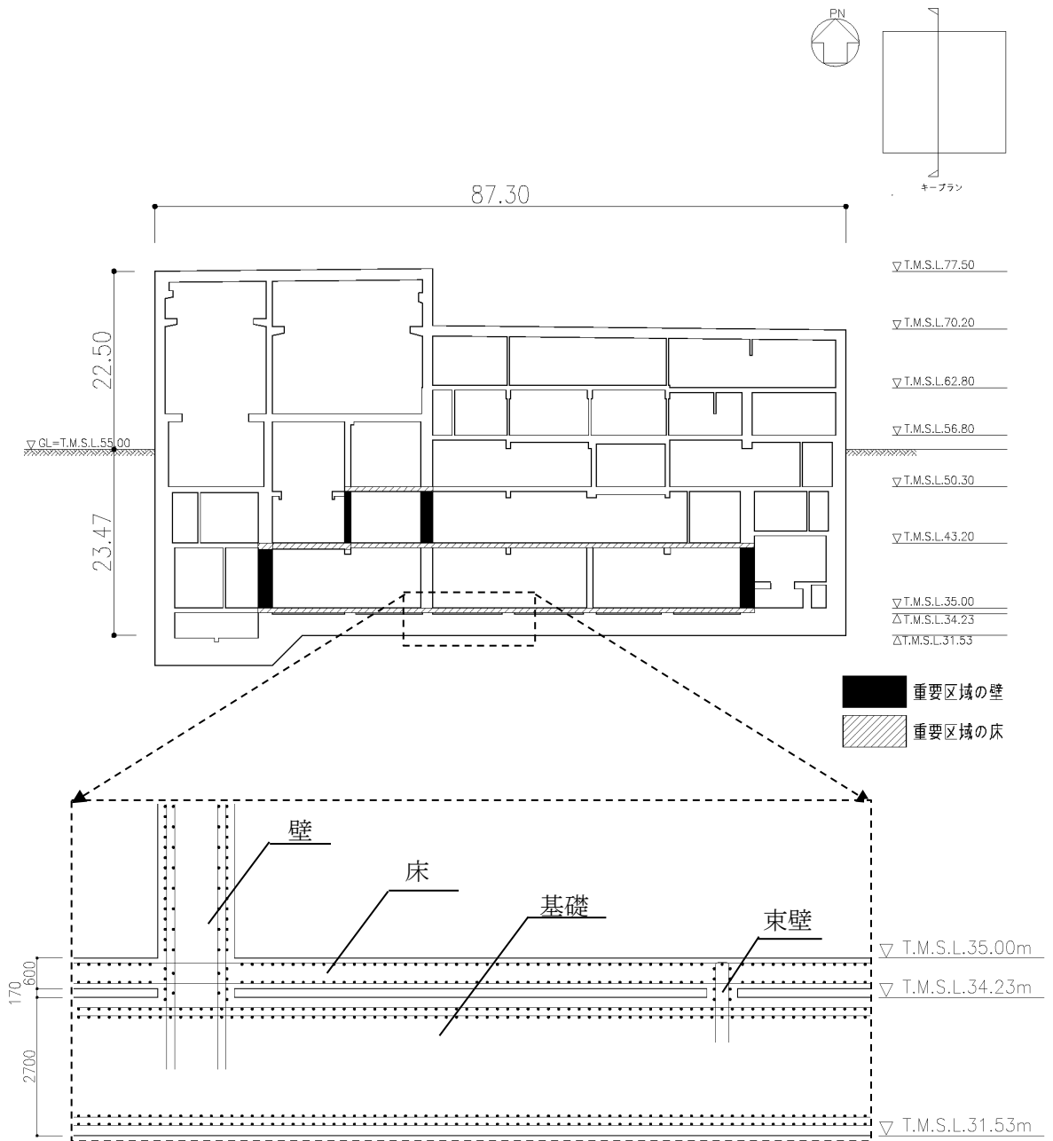
第 3-1 図 二重床部の詳細断面図
