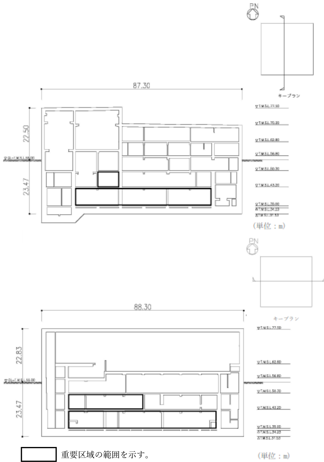
第 3.2-2 図 重要区域の範囲 (燃料加工建屋の概略断面図) 【上：NS 方向，下：EW 方向】
