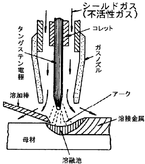
Tig 溶接
