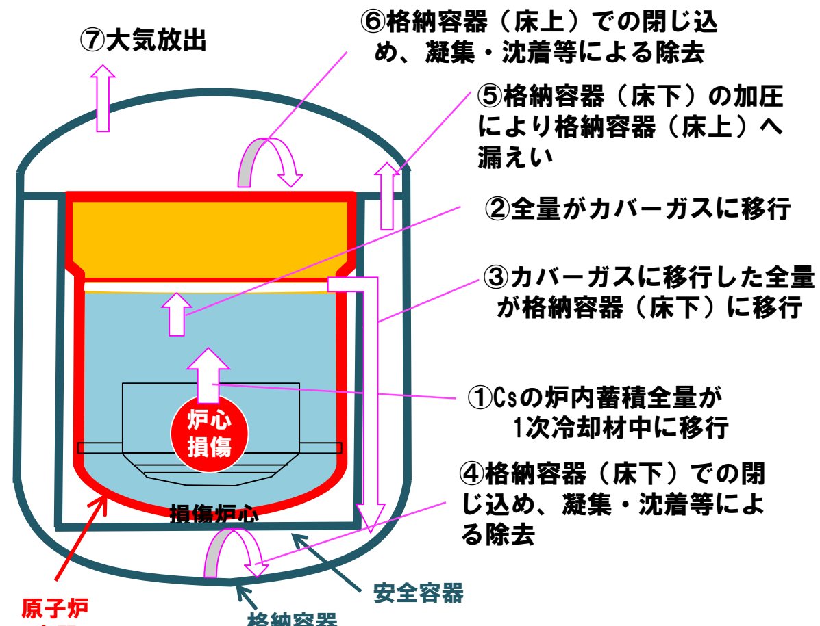
崩壊熱除去機能喪失型の評価の概念図
