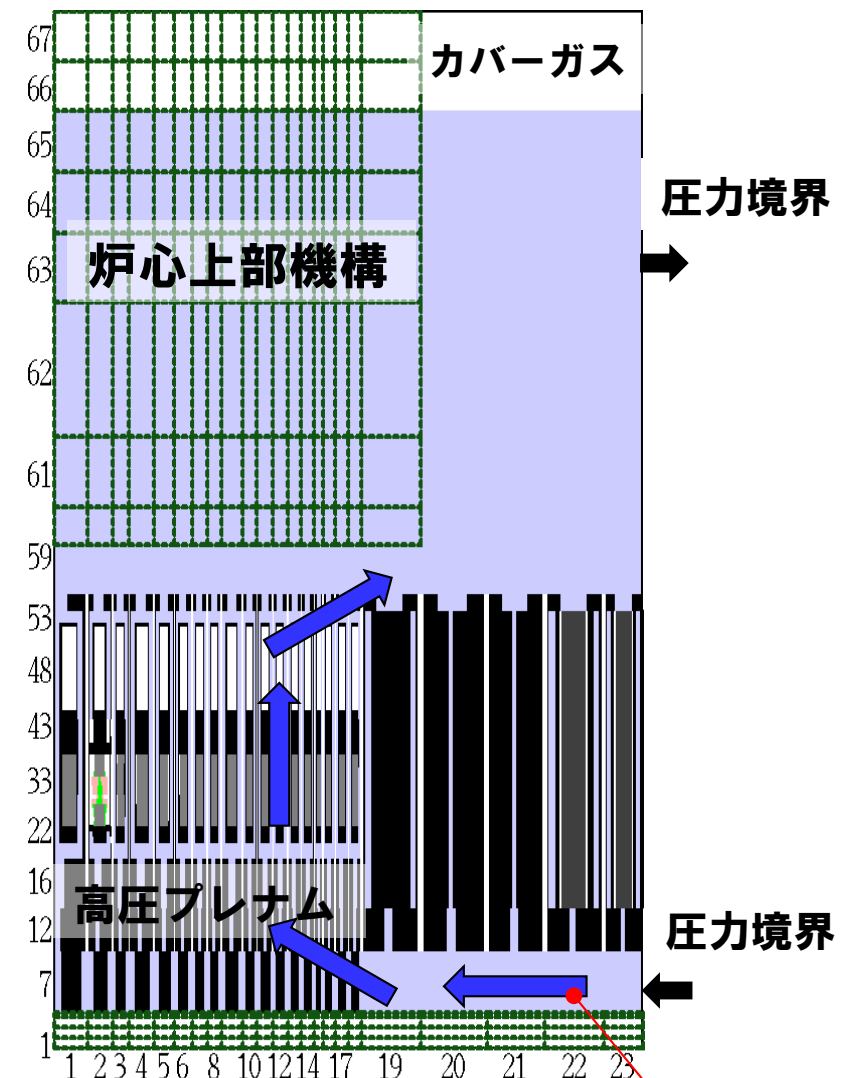
SIMMER-IIIの解析体系図
