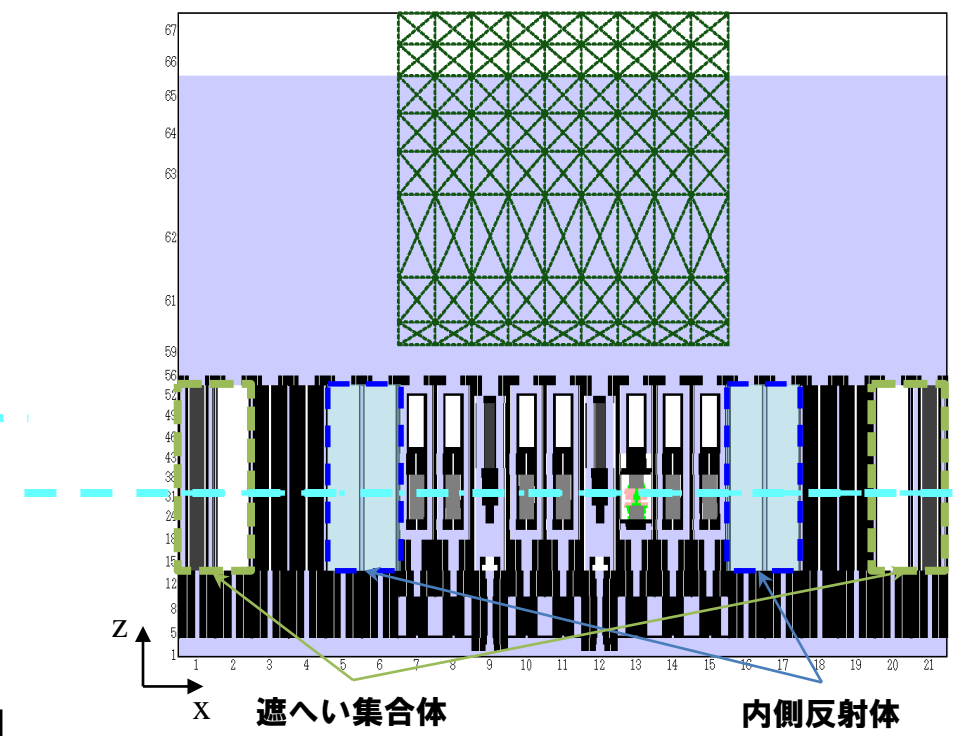
SIMMER-IVの解析体系: 炉心鉛直断面図
