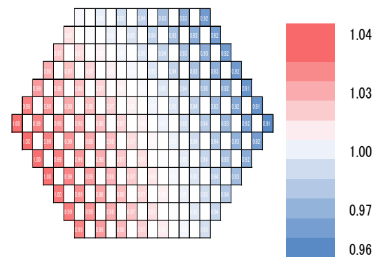
径方向出力分布
