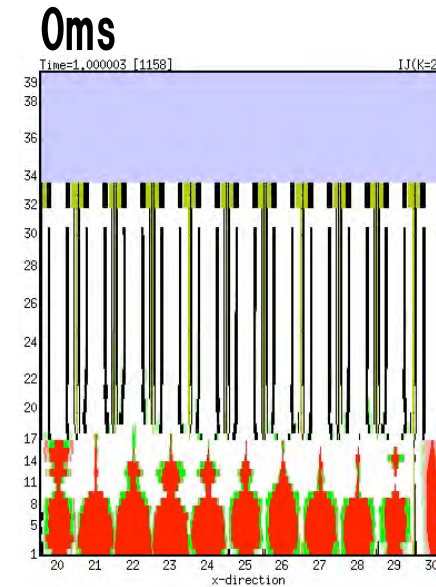
反射体ペレット削除ケース
