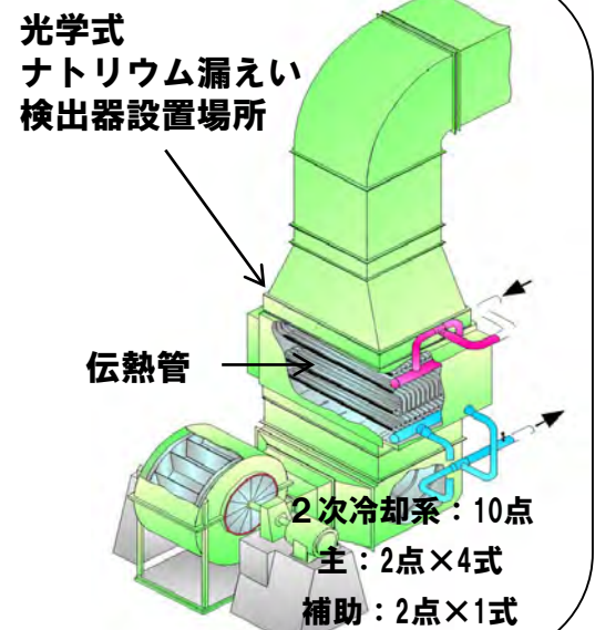
主冷却機（フィン付空冷多管式）
