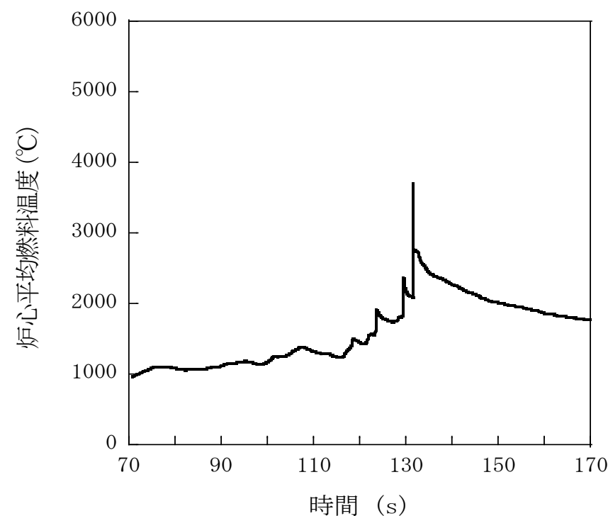
炉心平均燃料温度の推移
