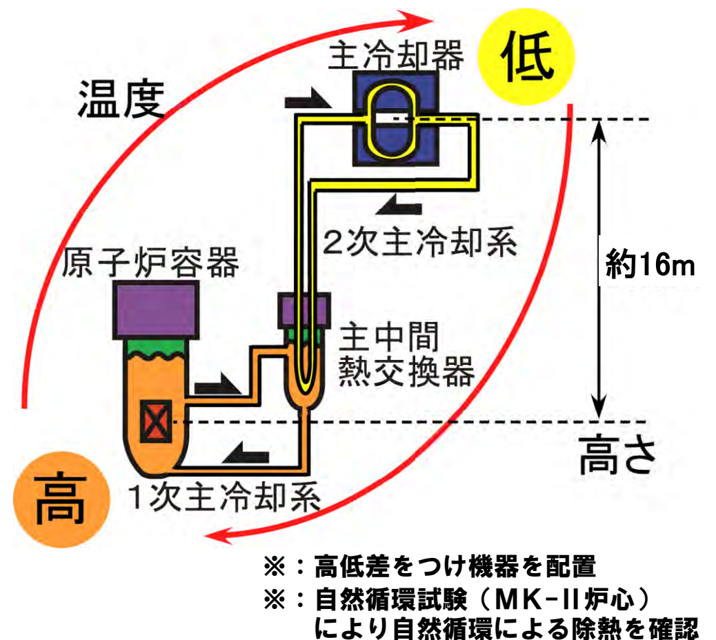
自然循環の概念図
