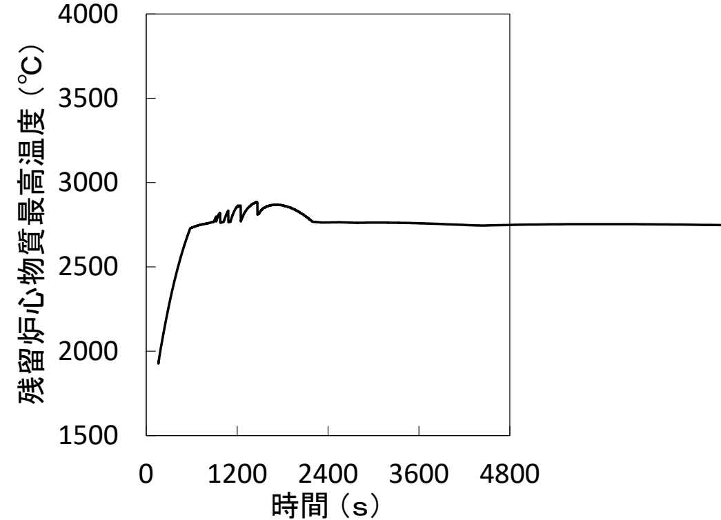
残留炉心物質最高温度の履歴
