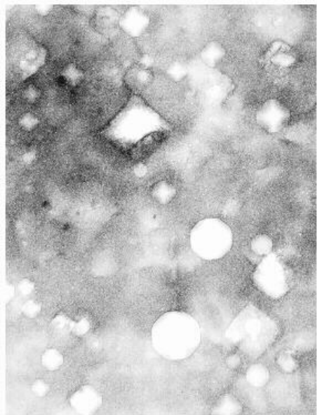
Ni, 37dpa
