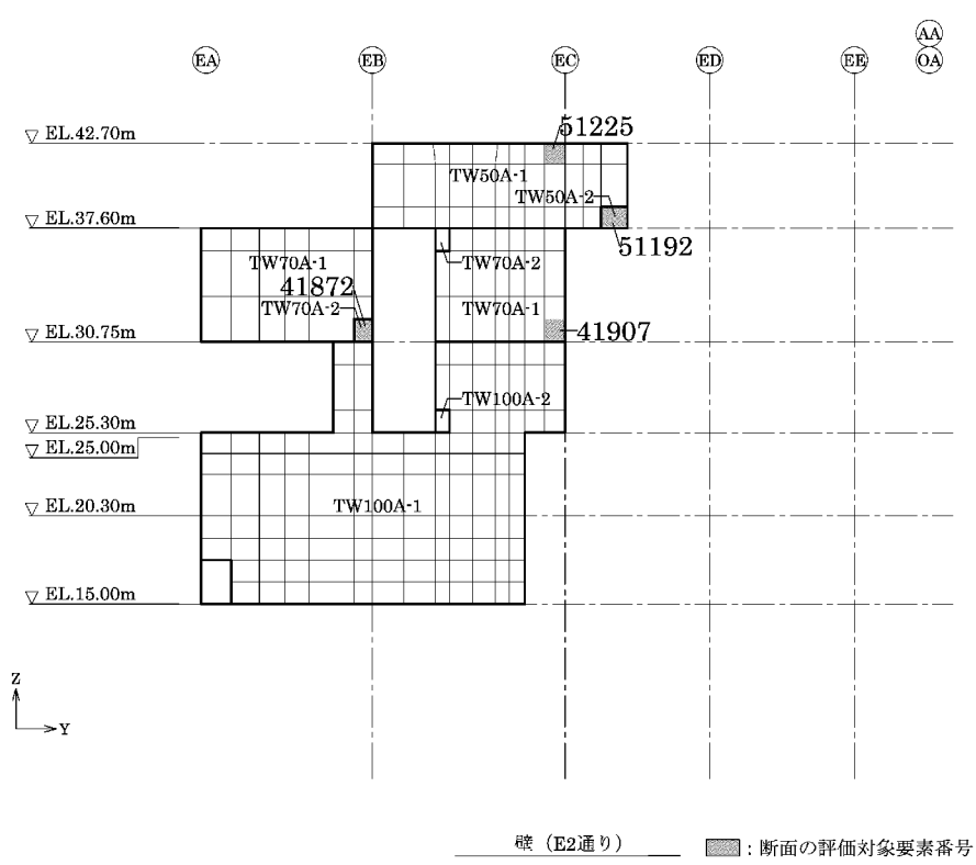
第 2-1 図 断面の評価対象要素番号(1/13)
