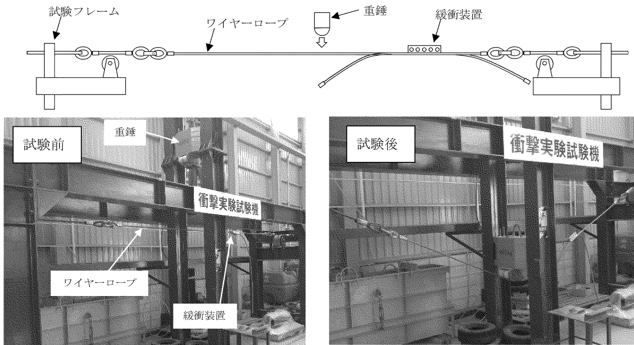
図1 実験設備概要
