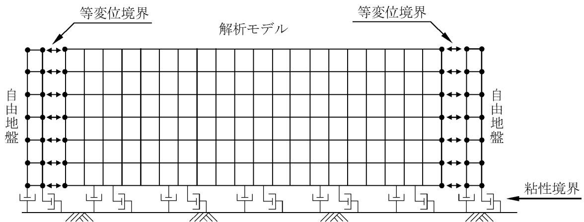
第 2-7 図 地盤モデルの境界条件概念図
