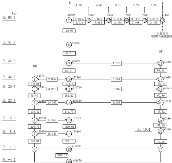
鉛直モデル
