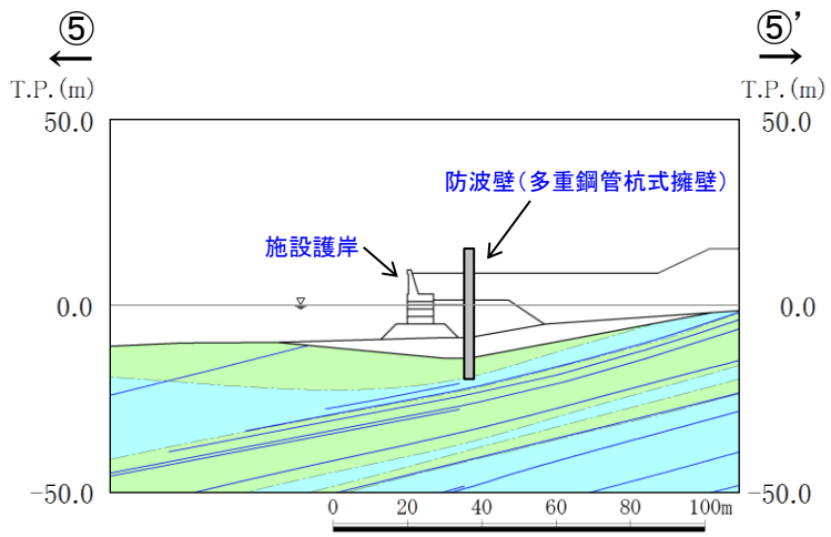
⑤-⑤' 断面図
