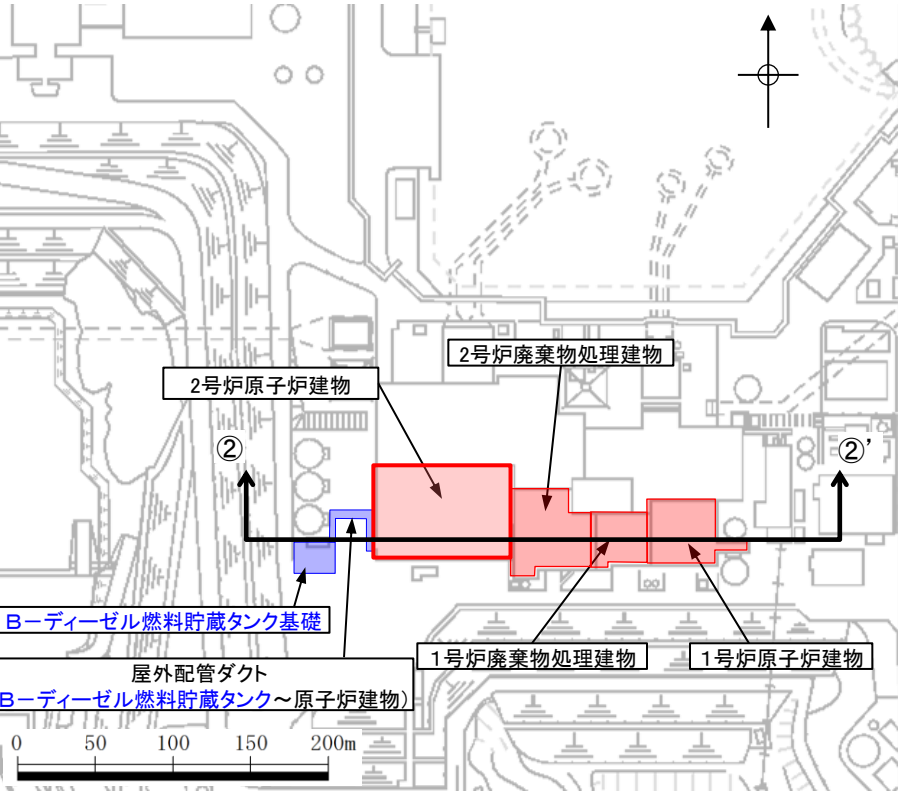
断面位置図
