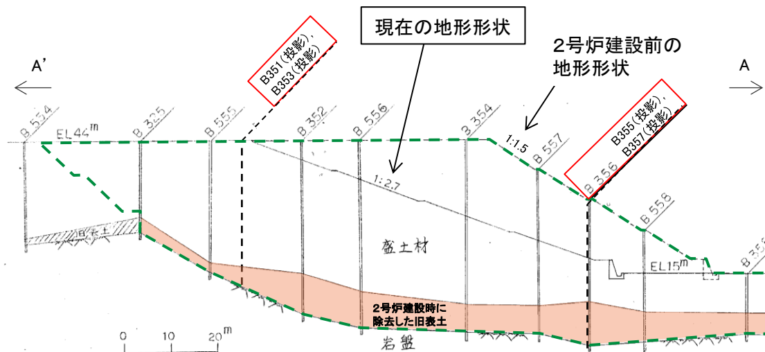
断面図(A-A' 断面)
