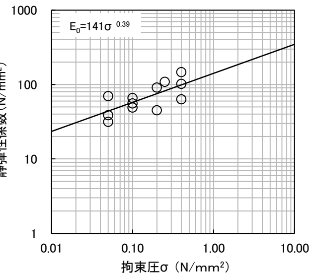
三軸圧縮試験結果 (凝灰岩・凝灰角礫岩)
