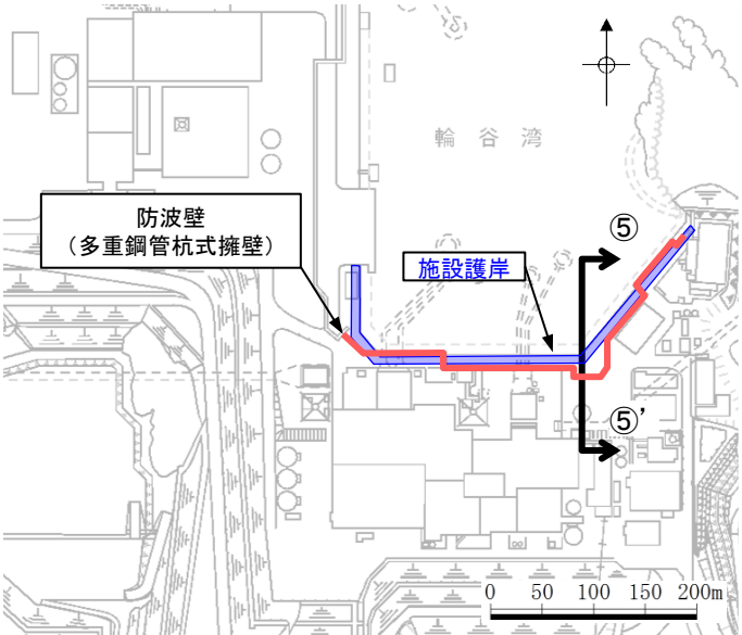
断面位置図
