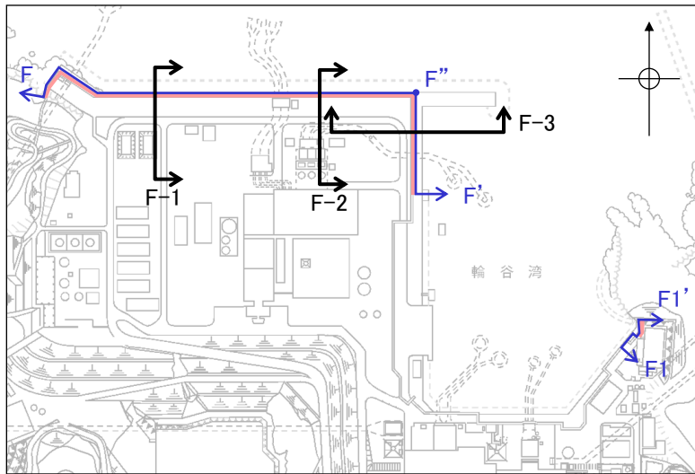
断面位置図
