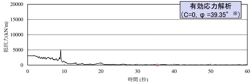
有効応力解析における埋戻土内のすべり面上の抵抗力 (Ss-D(-, -)) ※FLIPのせん断強度、「防波壁の構造成立性」の審査において設定した値(P183参照)
