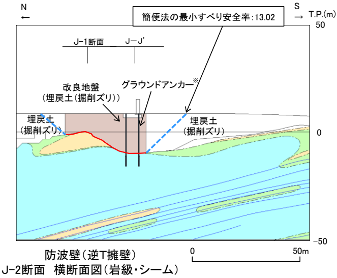
J-2断面 簡便法の結果
