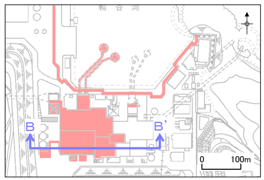
断面位置図 ■ : 評価対象施設
