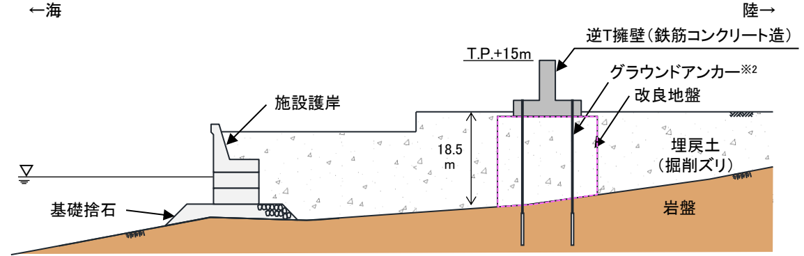
防波壁(逆T擁壁)鉛直断面図※1
