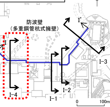
断面位置図
