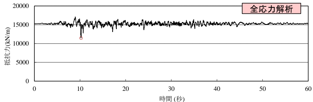
全応力解析における埋戻土内のすべり面上の抵抗力 (Ss-D(-, -))
