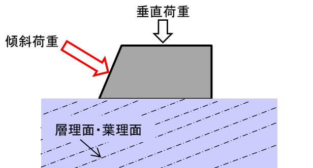
層理・葉理に沿う方向 (流れ目方向)の試験
