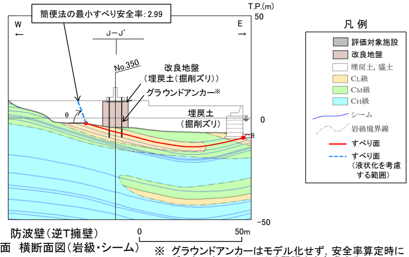
J-3断面 簡便法の結果
