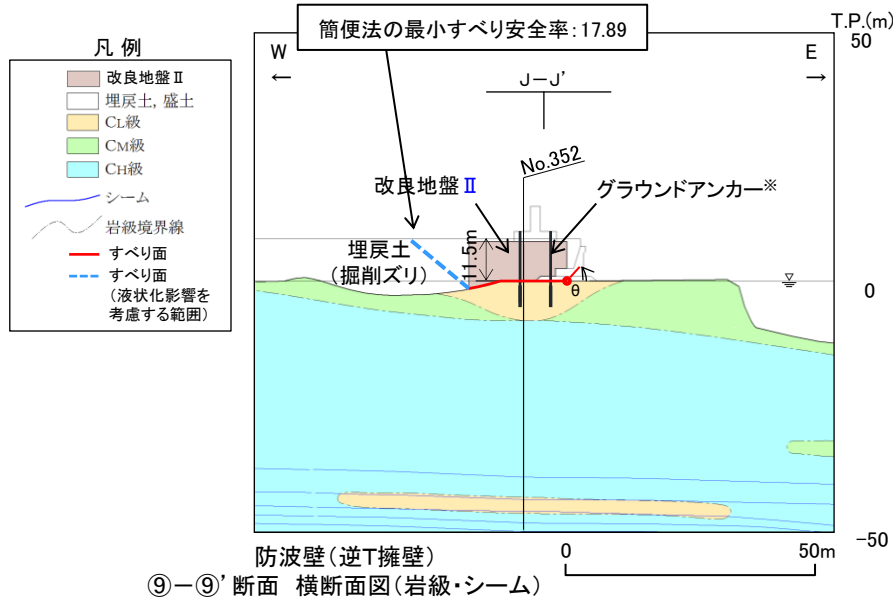
防波壁(逆T擁壁) 縦断面図(岩級・シーム)
