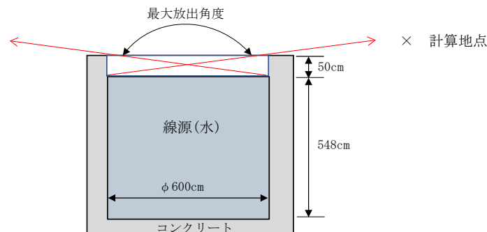
第 6 図 ANISN-G33 計算モデル
