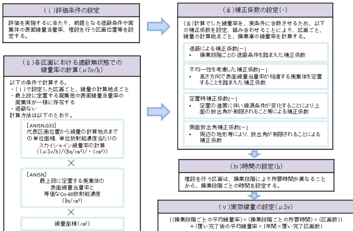
第7図 線量評価の流れ(埋設する放射性廃棄物の受入れの開始から覆土完了までの間)
