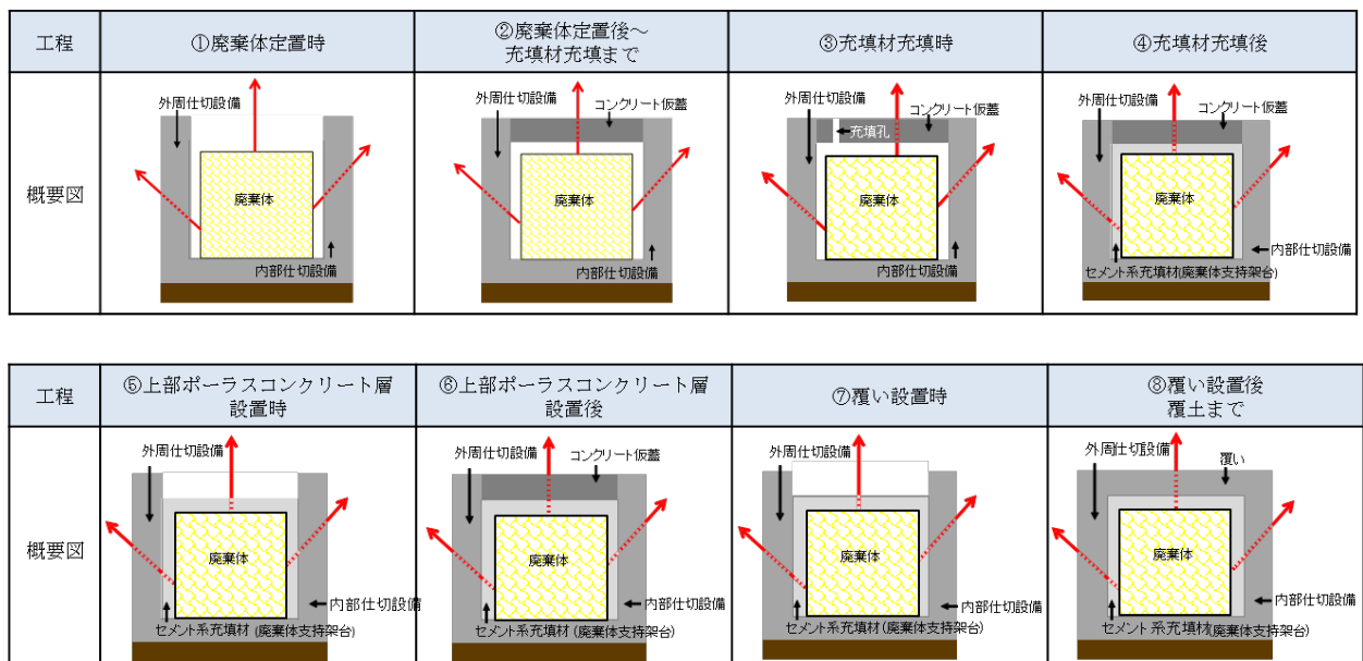
第1図 操業段階ごとの遮蔽の状況
