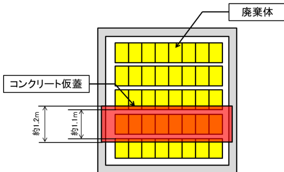
第7図 埋設クレーンによるコンクリート仮蓋の取付け・取外し時の操作員の誤操作における 損傷廃棄体イメージ平面図
