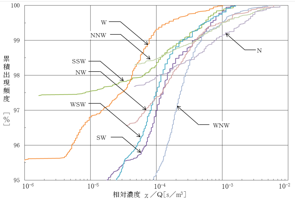
第11図 3号廃棄物埋設地放出の方位別相対濃度の累積出現頻度(1/2)
