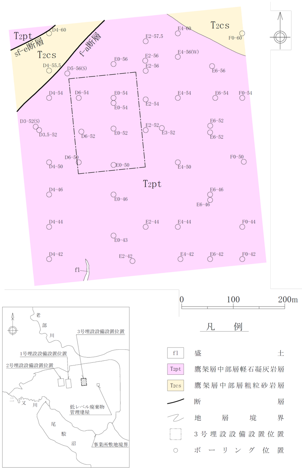
第 5 図 3 号廃棄物埋設地及びその付近の地質水平断面図(標高 22m)
