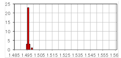
B4-57孔 GL-1.55m (Toya) ガラス屈折率頻度分布図
