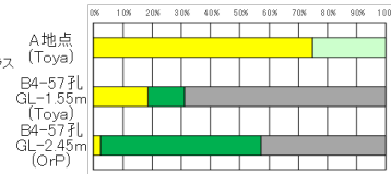
重鉱物組成分析結果
