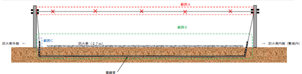
第3-3図 防火帯を横断しているケーブルの例
