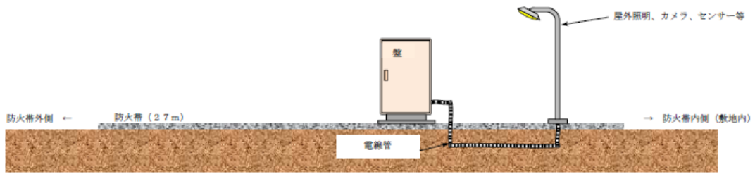
第3-1図 防火帯内に設置されている設備・機器等の例
