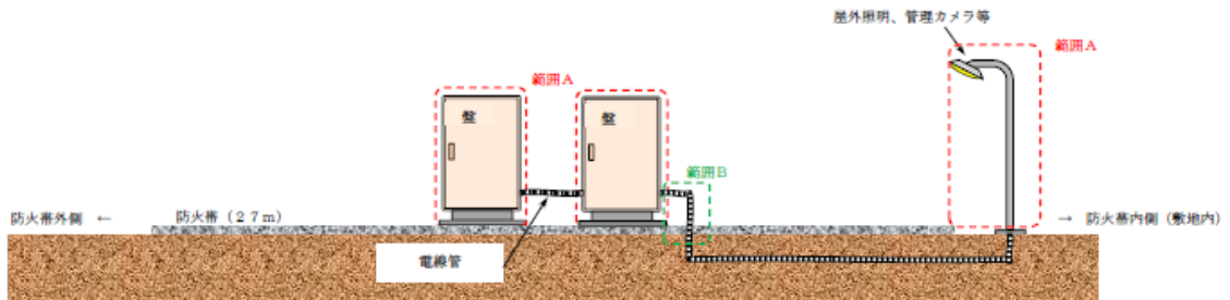
第3-2図 防火帯を横断している設備・機器等の例
