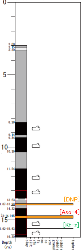
孔名: S-4(EL=333.455m)
