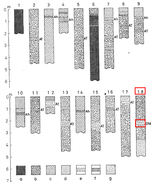
第5図 柱状図
