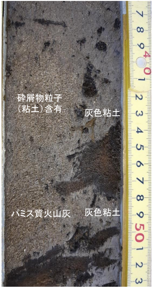
コア半割拡大写真(12.4m付近)
