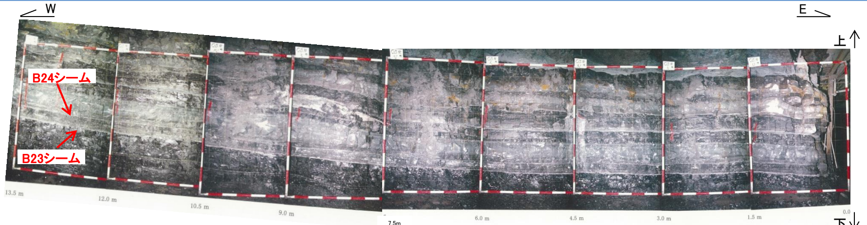
試掘坑側壁写真(北壁)
