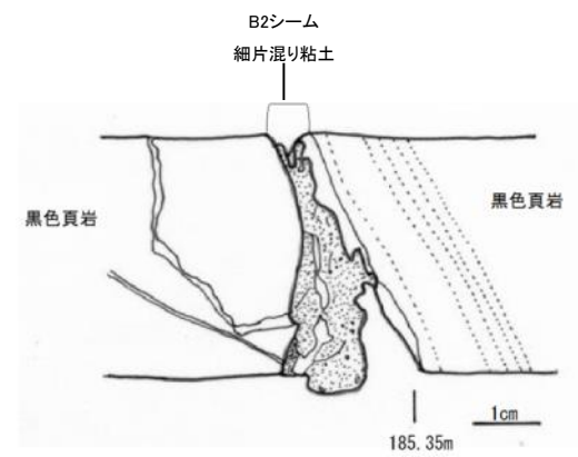
背斜軸南側のボーリング結果の例(No.B-4)
