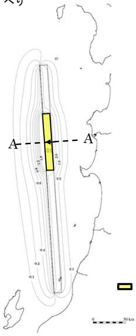
地盤変動量分布図
