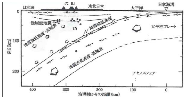
図 3.6 東北日本の地殻・上部マントルの東西鉛直断面模式図 (Hasegawa et al., 1994)
