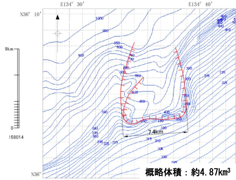
海底地形図 (日本水路協会(2008a)に加筆)
