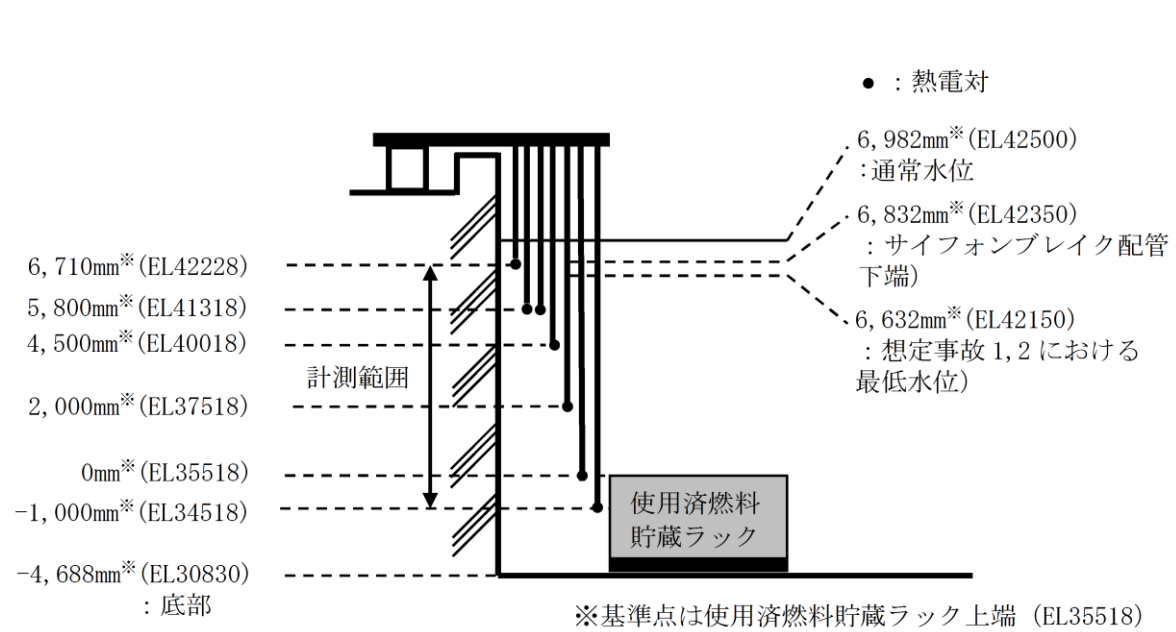
図3 燃料プール水位・温度 (SA) の設置図
