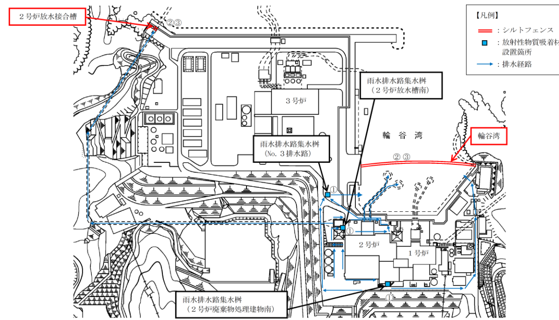
図 6-2 放射性物質吸着材及びシルトフェンスの設置位置図
