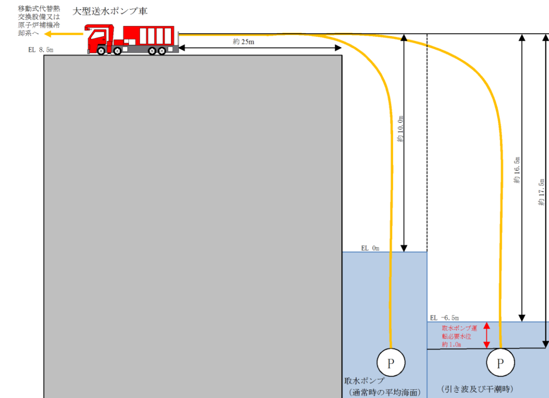
図13 大型送水ポンプ車概要図
