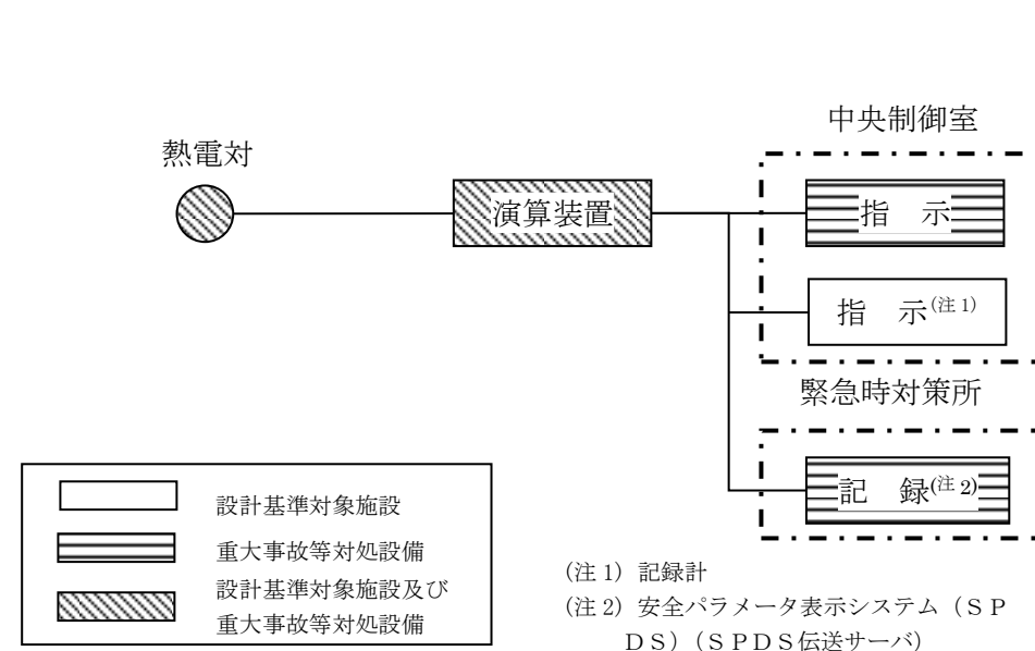
図2 燃料プール水位・温度 (SA) の概略構成図 (2)
