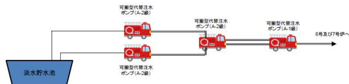
図5 燃料プール代替注水系 (常設スプレーヘッド) によるスプレー系統概要図
