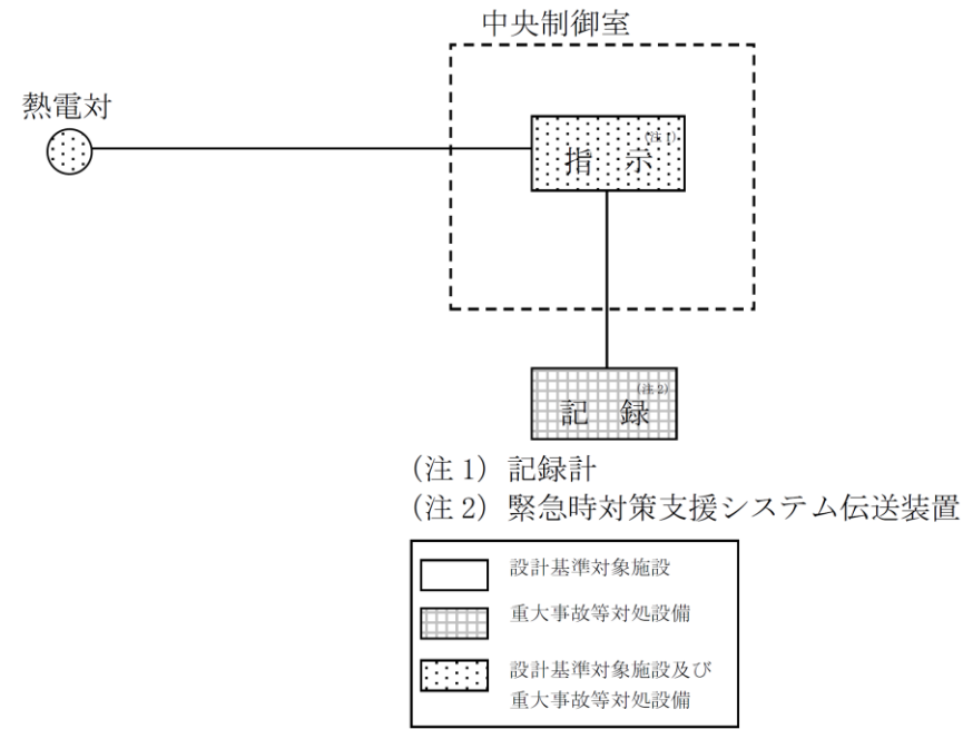
図2 使用済燃料貯蔵プール温度 (SA 広域) の概略構成図
