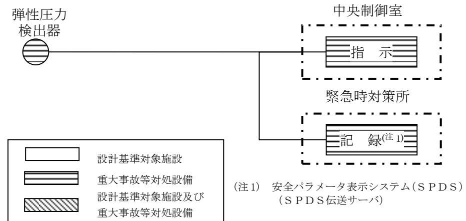
図2 スクラバ容器圧力の概略構成図
