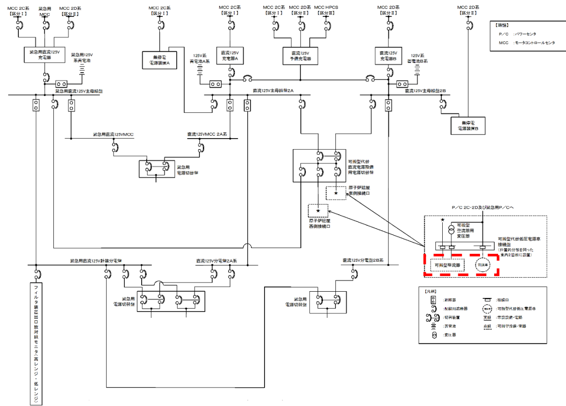
第6図 可搬型代替直圧電源設備による電源給電範囲
