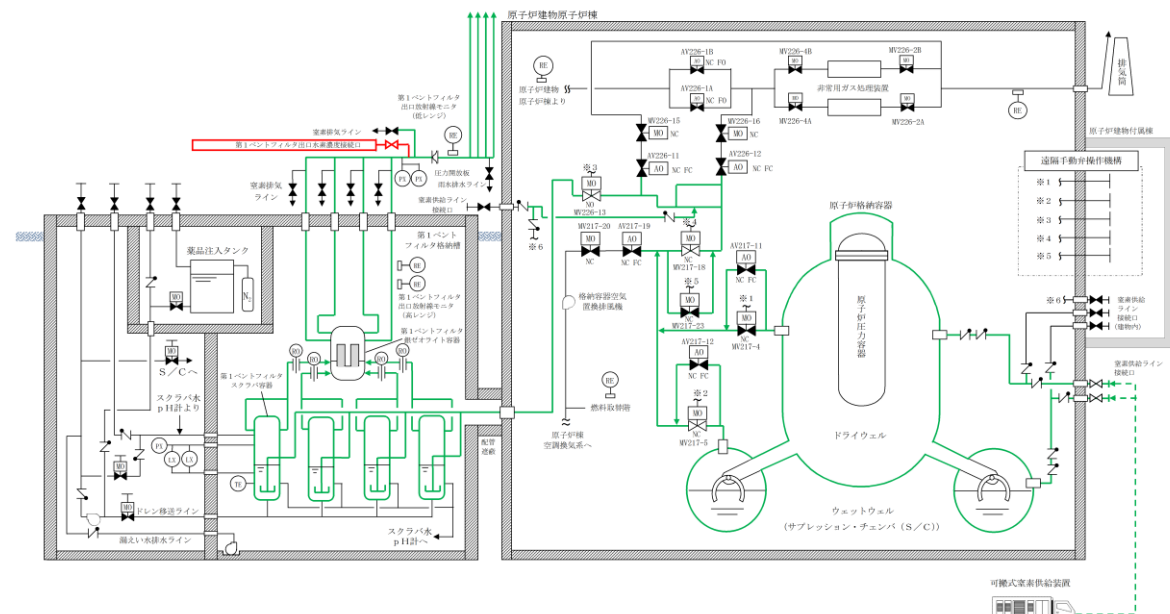
図 4.2.3-1 窒素供給及び水素濃度測定時の系統状態概要図
