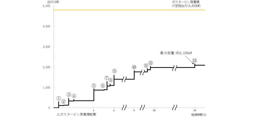
常設代替交流電源設備の負荷積算イメージ
