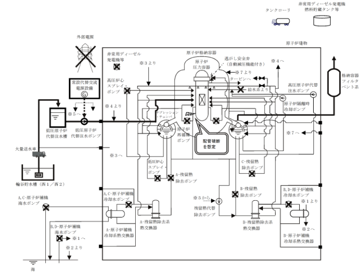
第 3.1.3.1-1(3) 図 「雰囲気圧力・温度による静的負荷 (格納容器過圧・過温破損)」の重大事故等対策の概略系統図 (残留熱代替除去系を使用しない場合) (原子炉注水及び原子炉格納容器除熱)
