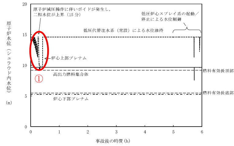
第2.7-5図 原子炉水位 (シュラウド内水位) の推移
