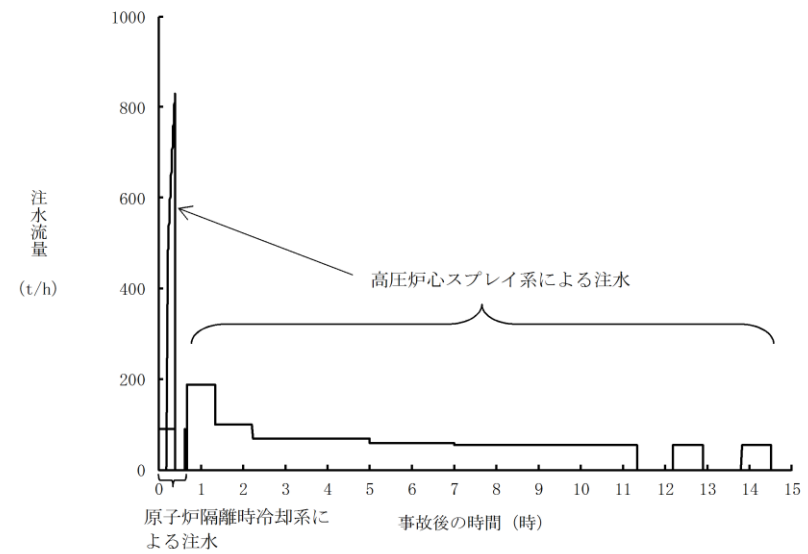
第 2.7.2-1(4) 図 注水流量の推移
