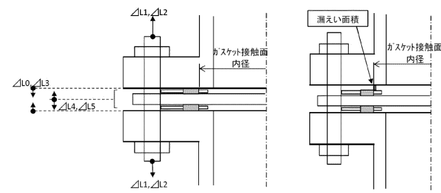
図 1-6 各部分材の伸び方向及び伸び時隙間想定位置
