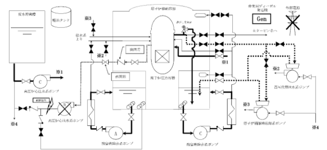
第2.7.2図 「格納容器バイパス(インターフェイスシステム LOCA)」の重大事故等対策の概略系統図(2/3) (原子炉注水及び原子炉格納容器除熱)
