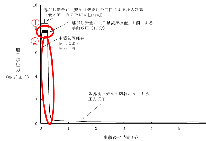
第 2.7-4 図 原子炉圧力の推移
