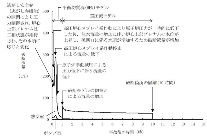
第 2.7.2-1(10) 図 破断流量の推移
