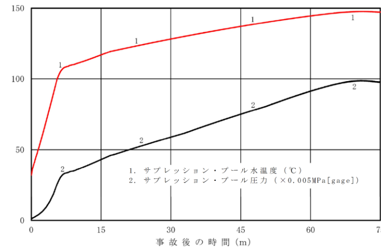
第12図 サプレッション・プール水温度及び格納容器圧力の推移 (長期)
