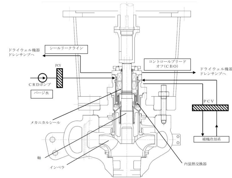
図1 PLRポンプ 概略図
