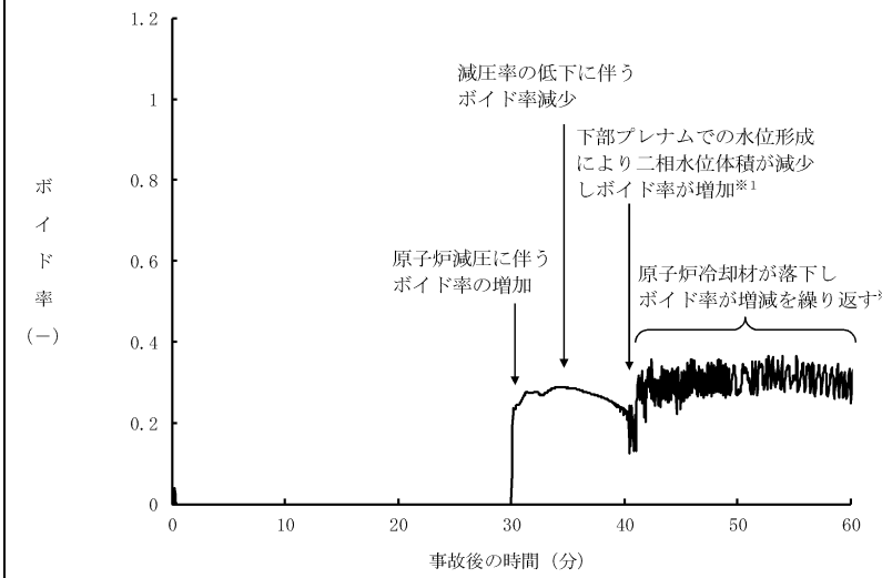
第 2.1.2-1(11)図 炉心下部プレナム部のボイド率の推移
