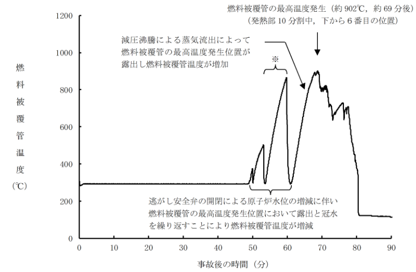
図4 操作開始時間 30分遅れの場合における燃料被覆管温度の推移
