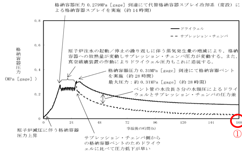
第 2.1-16 図 格納容器圧力の推移
