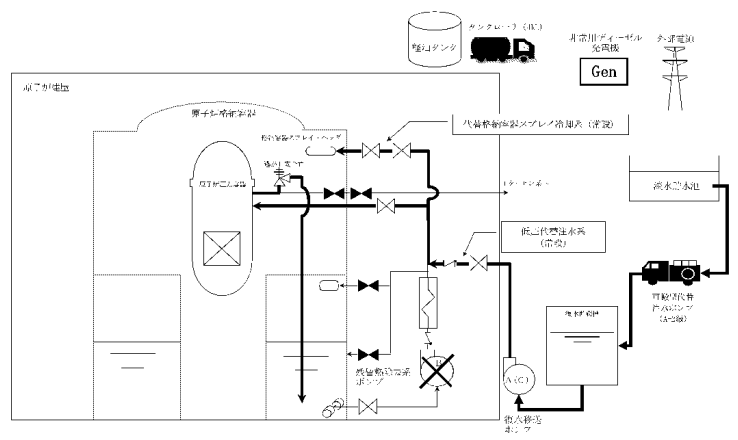
第 2.1.2 図 「高圧・低圧注水機能喪失」の重大事故等対策の概略系統図 (2/3) (原子炉注水及び原子炉格納容器冷却)
