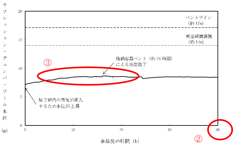
第 2.3.2.18 図 サプレッション・チェンバ・プール水位の推移
