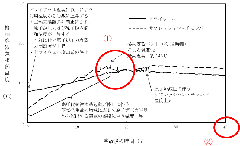
第 2.3.2.17 図 格納容器気相部温度の推移
