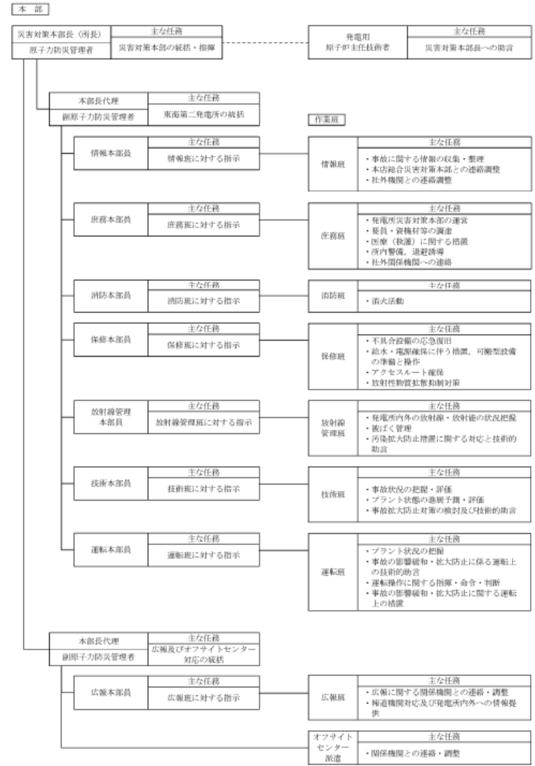
第2.1図 原子力防災組織 (東海第二発電所) (新規基準として申請している組織を示す)
