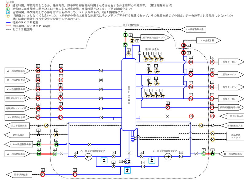
原子炉冷却材圧カバウンダリ図
