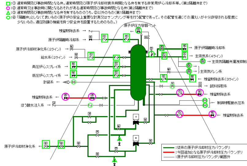
別 2-1 図 原子炉冷却材圧カバウンダリ概要図
