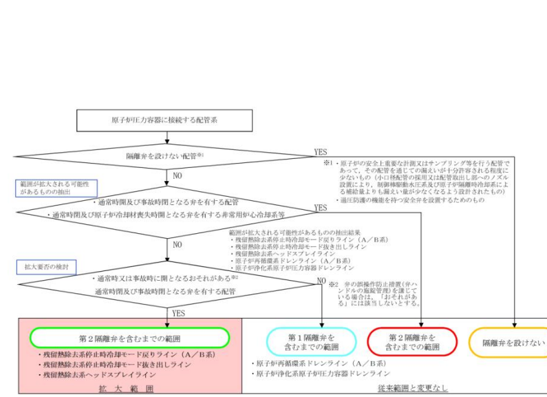
原子炉冷却材圧カバウンダリ弁抽出フロー
