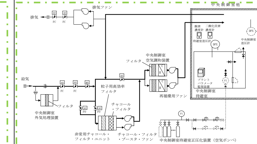
図 2.4-9 中央制御室換気系 機器概要図
