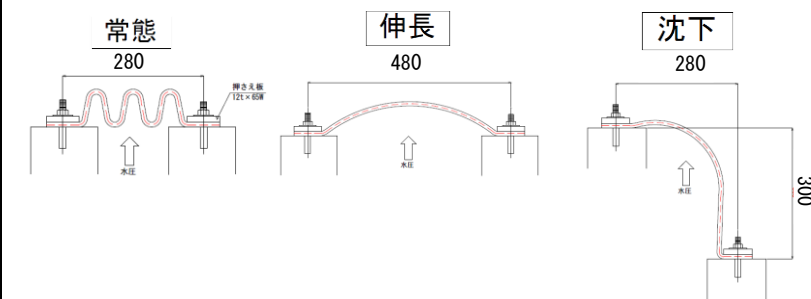
図2 止水板の耐水圧試験概略図
