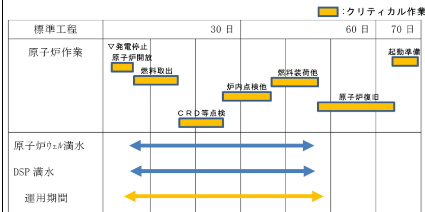
第 11 図 施設定期検査工程例
