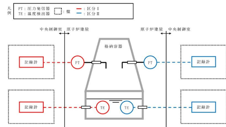
第 29-2 図 原子炉格納容器圧力計装, サプレッション・プール水温度計装 系統概略図
