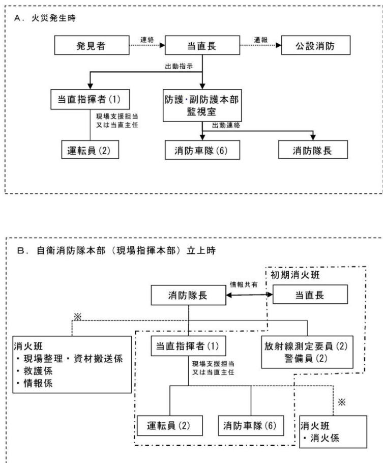
第 1-42 図 自衛消防隊編成（発電関連設備）
