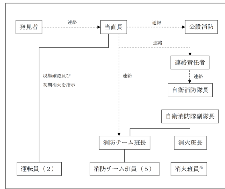
第 1-41 図 自衛消防隊編成（発電関連設備）
