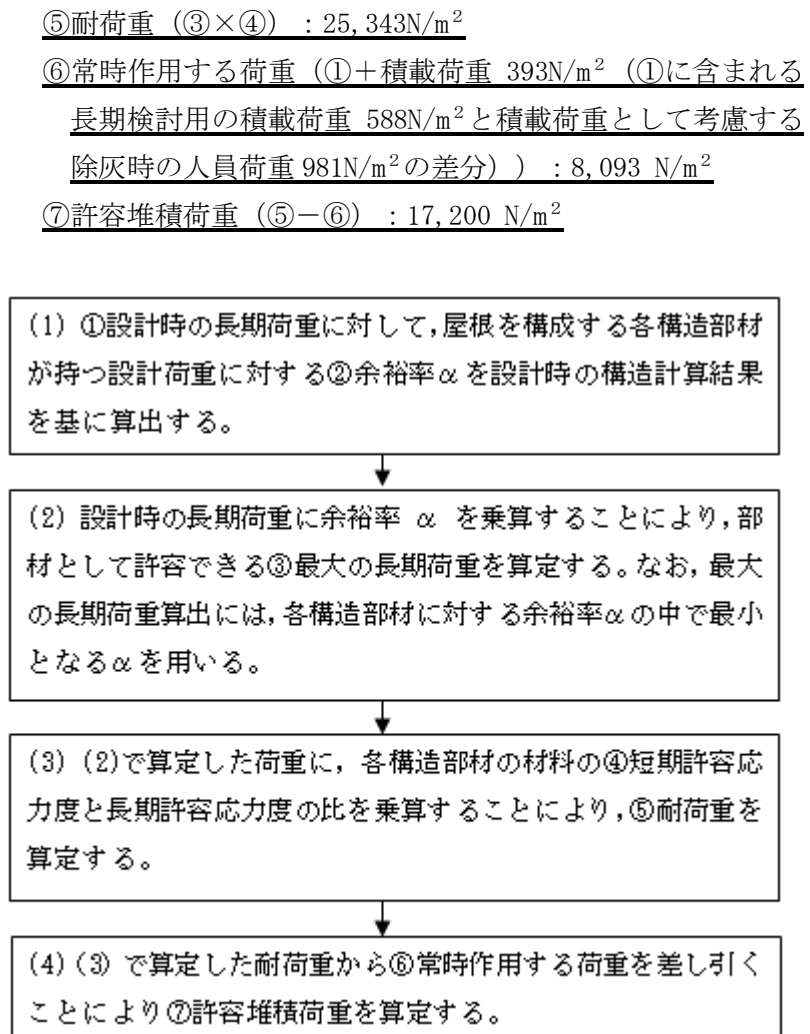
第1-3図 耐荷重算定フロー
