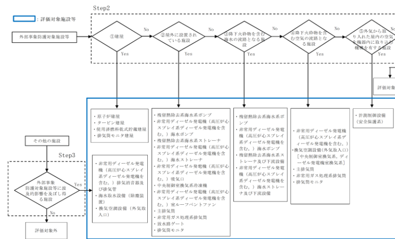
第 3.3-2 図 評価対象施設等の抽出フロー
